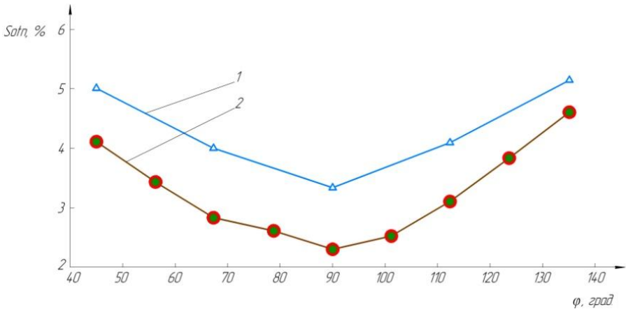
Рисунок 2 – Відносна площа зрізу зерном при шліфуванні для реального нахилу зерен ( \beta ) в робочому шарі круга S_v , де 1 – графік зміни площі від кута нахилу для одного зерна, 2 – графік зміни площі від кута нахилу для 1000 зерен
