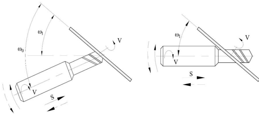
Рисунок 7 – Схема изменения ориентации осей заготовки сверла и шлифовального круга методом поворота оси шпинделя заготовки
