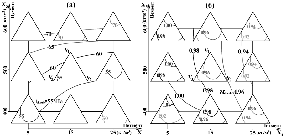
Рис.1. Влияние варьируемых факторов состава декоративных судостроительных бетонов на их прочность при сжатии (а) и относительное изменение прочности при сжатии \delta f_{k,cube} при введении пигментов (б)
