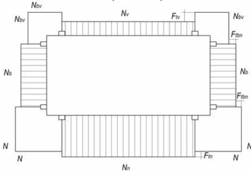
Рис. 3. Эпюра усилий по периметру обоймы
