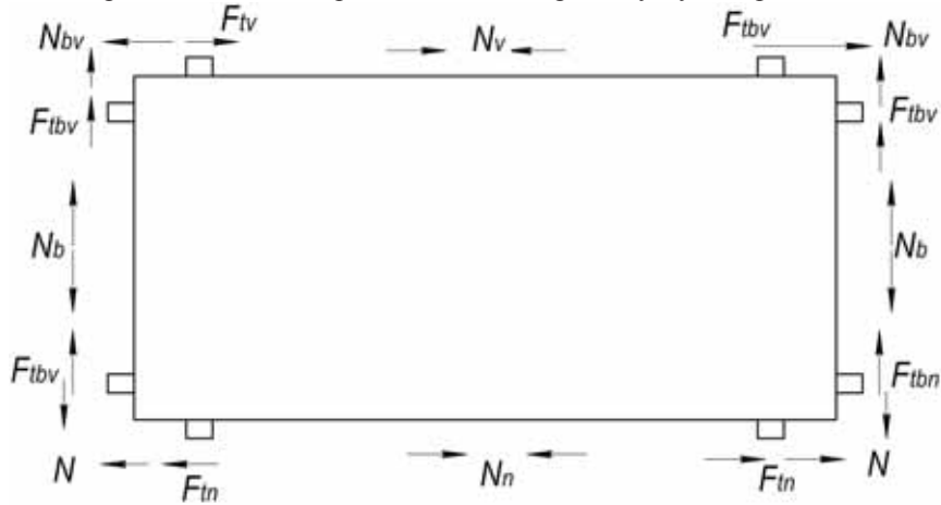
Рис. 2. Схема усилий в замкнутой обойме
