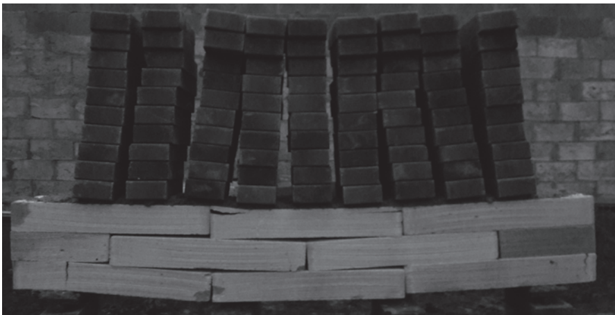
Рис. 7. Разрушение образца из трех слоев блоков без раствора
