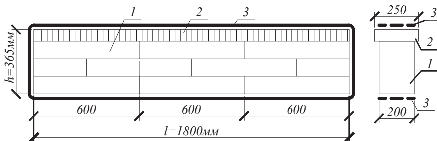
Рис. 3. Конструкция комбинированной перемычки из газоблоков и кирпича 5) - из трех рядов газобетонных блоков толщиной 100 мм (размеры 600x200x100 мм) с перевязкой швов без раствора (см. рис. 2). Обойма из трех замкнутых элементов (см. рис. 1-3) из полипропиленовой упаковочной ленты: размеры сечения 18.85x0.94 мм; разрывное усилие – 2.79 кН.
