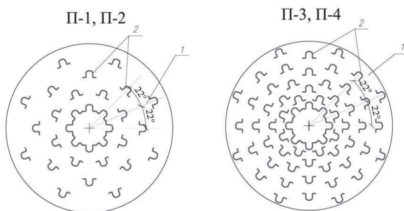
Рис. 1. Сталебетонные круглые плиты
