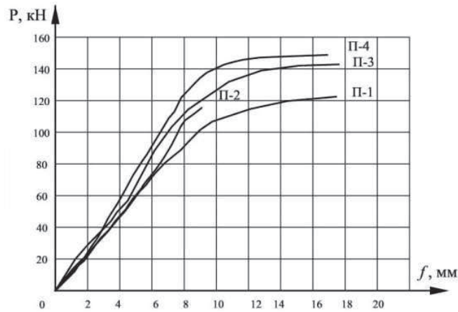
Рис. 5. Экспериментальные кривые прогибов для круглых плит
