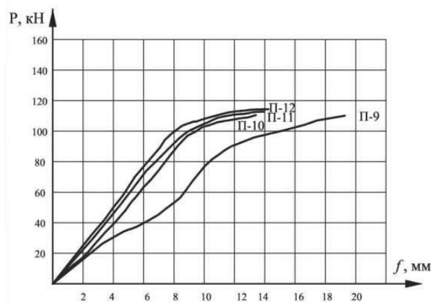
Рис. 7. Экспериментальные кривые прогибов для квадратных плит
