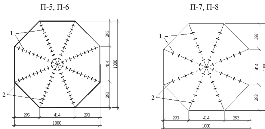
Рис. 2. Сталебетонные восьмиугольные плиты
