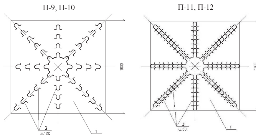
Рис. 3. Сталобетонные квадратные плиты
