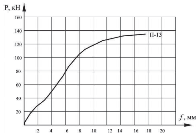
Рис.8. Экспериментальные кривые прогибов для квадратных плит с просечками
