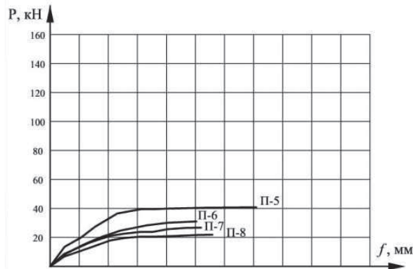
Рис. 6. Экспериментальные кривые прогибов для восьмиугольных плит
