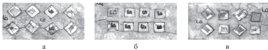
Рис.4. Вплив параметрів макроструктури на міцність та руйнування моделей бетонних зразків: а – f_{ck}=8,6 МПа; б – f_{ck}=9,4 МПа; в – f_{ck}=13,7 МПа.
