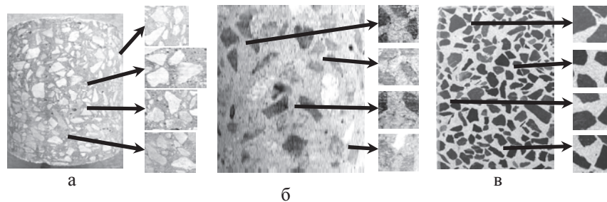
Рис.1. Різноманітність геометричних параметрів структурних чарунків у зразках-кернях реальних конструкцій: а – опорна стіна гідропоруди; б – залізобетонна; в – тротуарна плитка.
