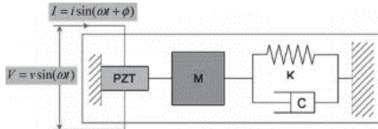
Рис. 2. Ідеалізована система електронного механізму
