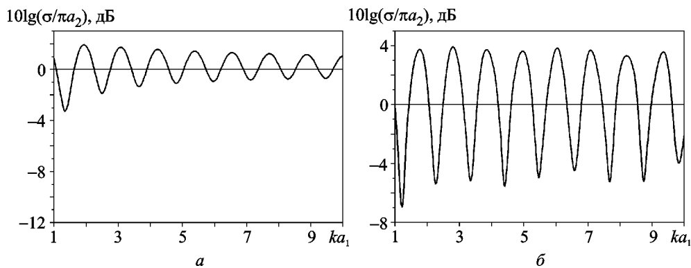
Рис. 5. Нормированное сечение обратного рассеяния проводящего цилиндра с диэлектрическим покрытием ( \epsilon = 4 ) для случая H -волны: a – h = 0.04\lambda , b – h = 0.1\lambda
