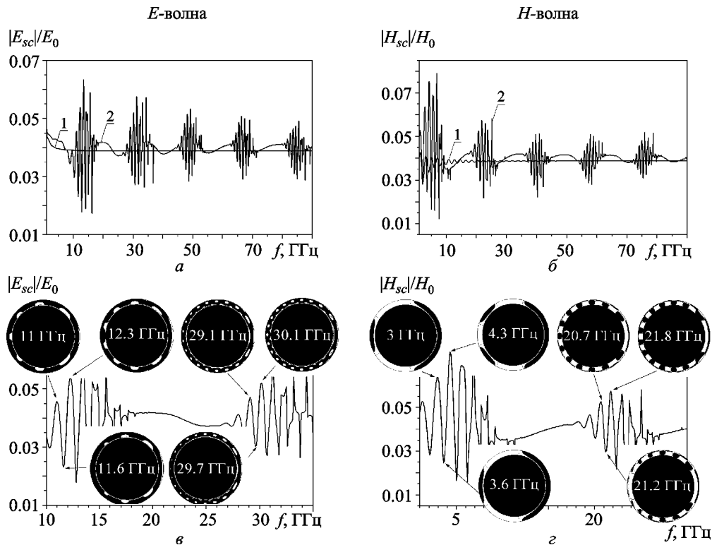
Рис. 2. Зависимость обратного ( \varphi = 0 ) рассеяния от частоты для E - и H -волны ( a и b ): кривая 1 – металлический цилиндр, кривая 2 – металлический цилиндр со слоем диэлектрика. Пространственные распределения \text{Re}\{H_\varphi\} и \text{Re}\{E_\varphi\} на частотах экстремумов – круговые черно-белые диаграммы ( v и z соответственно)
