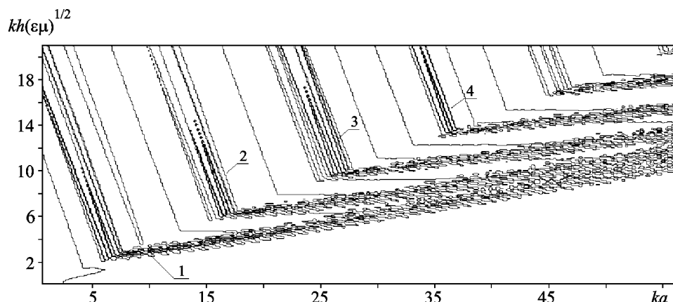
Рис. 4. Распределение рассеянного поля при изменении частоты и диэлектрической проницаемости слоя диэлектрика для случая E -волны
