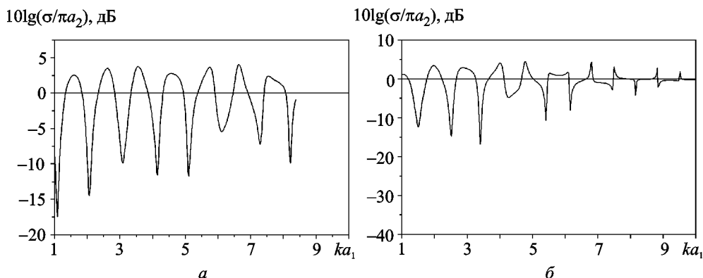
Рис. 6. Нормированное сечение обратного рассеяния проводящего цилиндра с диэлектрическим покрытием ( \epsilon = 2.56 , h = 0.41\lambda ): a – для случая E -волны, b – для случая H -волны
