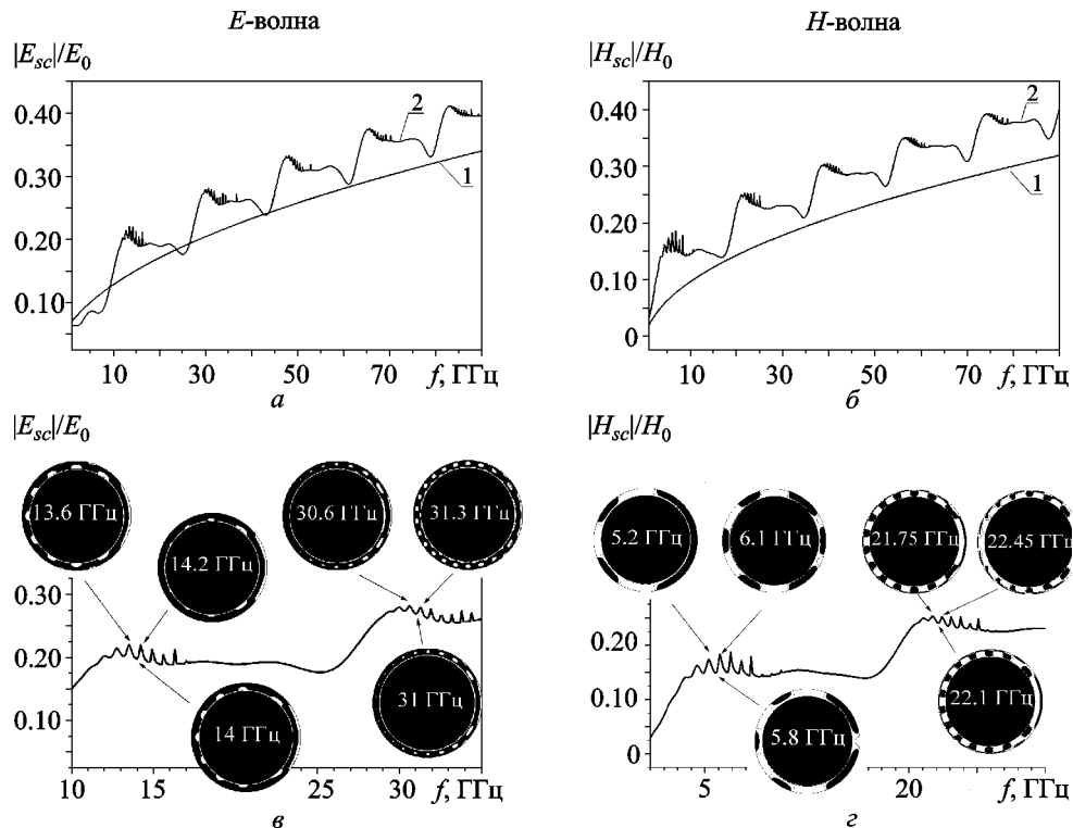
Рис. 3. Зависимость прямого ( \varphi = 180^\circ ) рассеяния от частоты для E - и H -волны (а и б): кривая 1 – металлический цилиндр, кривая 2 – металлический цилиндр со слоем диэлектрика. Пространственные распределения Re\{H_\varphi\} и Re\{E_\varphi\} на частотах экстремумов – круговые черно-белые диаграммы (в и з соответственно)
