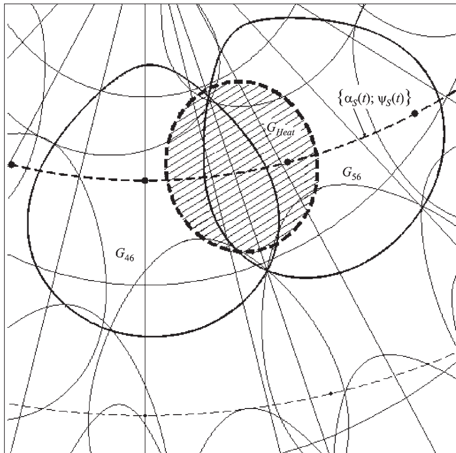
Рис. 3. Взаимное пересечение лучей (4;6), (5;6) риометра Гакона по уровню G_{mn}(\alpha, \psi) = 0 и главного лепестка нагревного стенда HAARP по уровню G_{Heat}(\alpha, \psi) = 0.5 (штриховая окружность) в наблюдениях 13. 11. 2012 г.
