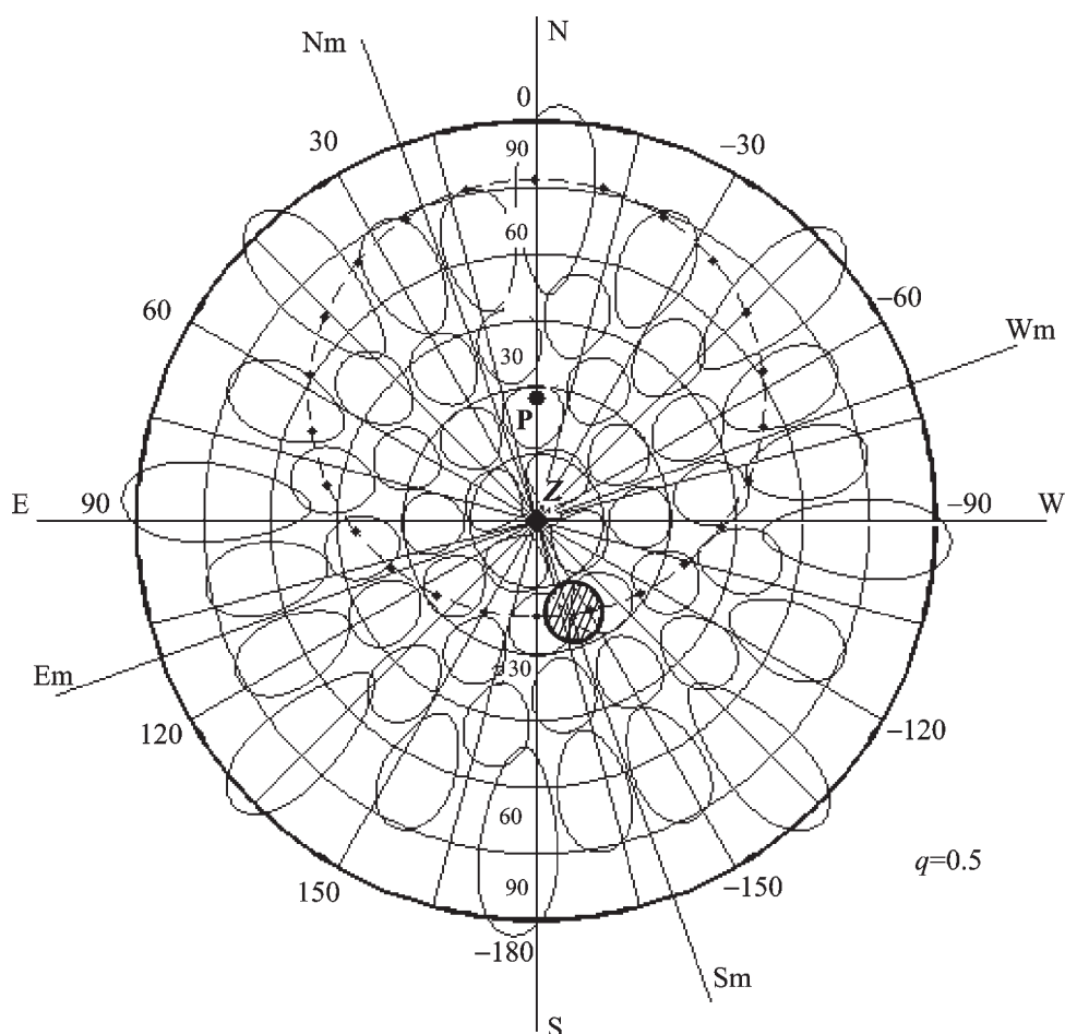
Рис. 1. Диаграмма направленности риометра Гакона: штрих-пунктирная окружность – траектория движения ДКИ Лебедь А, окружность с наклонной штриховкой – ориентация главного лепестка стелды HAARP в наблюдениях 13.11.2012 г.
