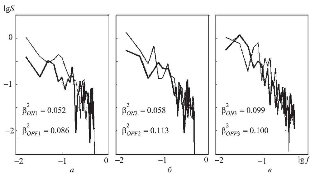
Рис. 4. Спектры и индексы мерцаний ДКИ Лебедь А в трех циклах нагрева 13.11.2012 г.: жирные линии – интервалы ON, тонкие – интервалы OFF
