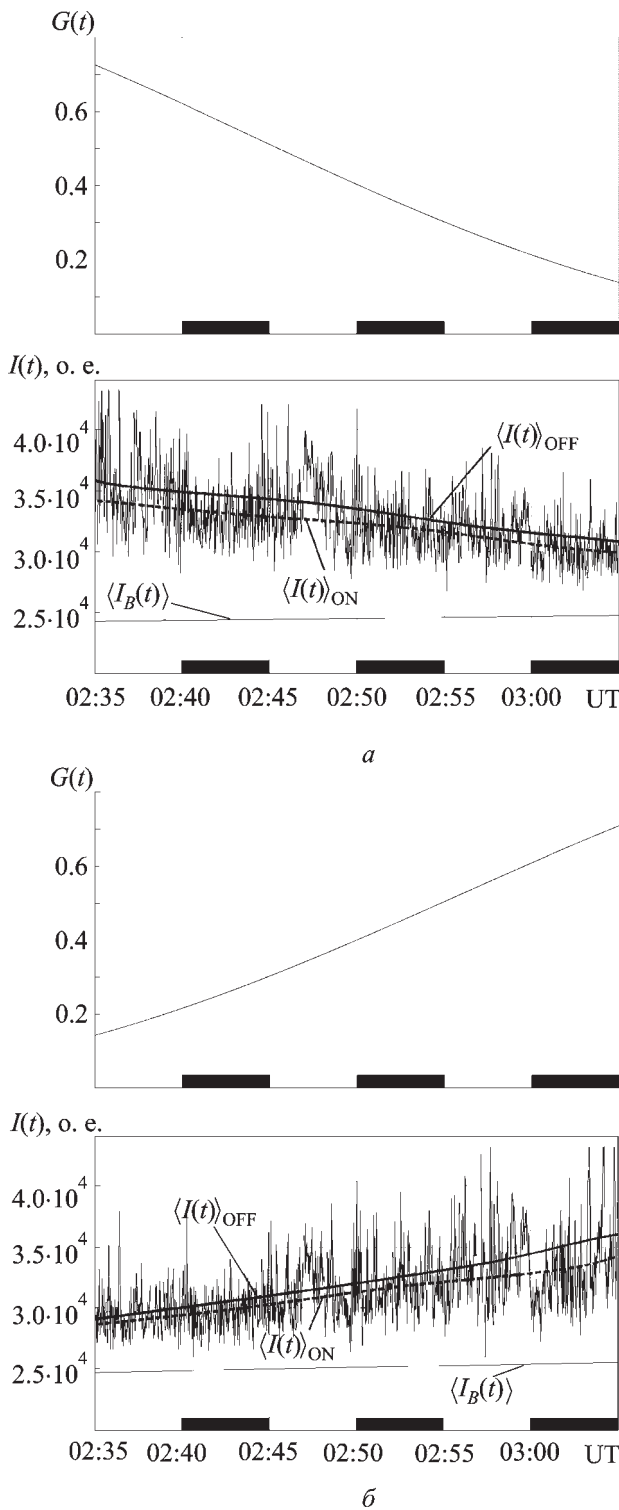
Рис. 2. Результаты первичной обработки данных: а – луч (4;6); б – луч (5;6). Темные прямоугольники вдоль оси абсцисс – интервалы включения нагревного стенда. Верхние панели рисунков – текущие значения расчетных диаграмм лучей (4;6), (5;6) риометра Гакона в направлении \{\alpha_S(t); \psi_S(t)\} на источник
