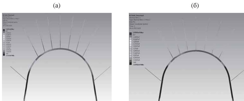
Рис. 2. Эпюры вертикальных напряжений \sigma_y рамной и анкерной крепи: при расстоянии 14 м от груди очистного забоя до выработки (а); грудь очистного забоя сравнялась с вертикальной осью симметрии выработки (б)
