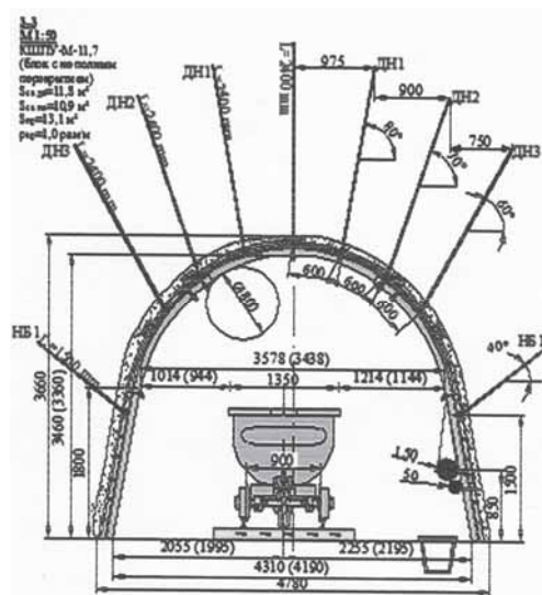
Рис.1. Схема рамного и анкерного крепления выработки
