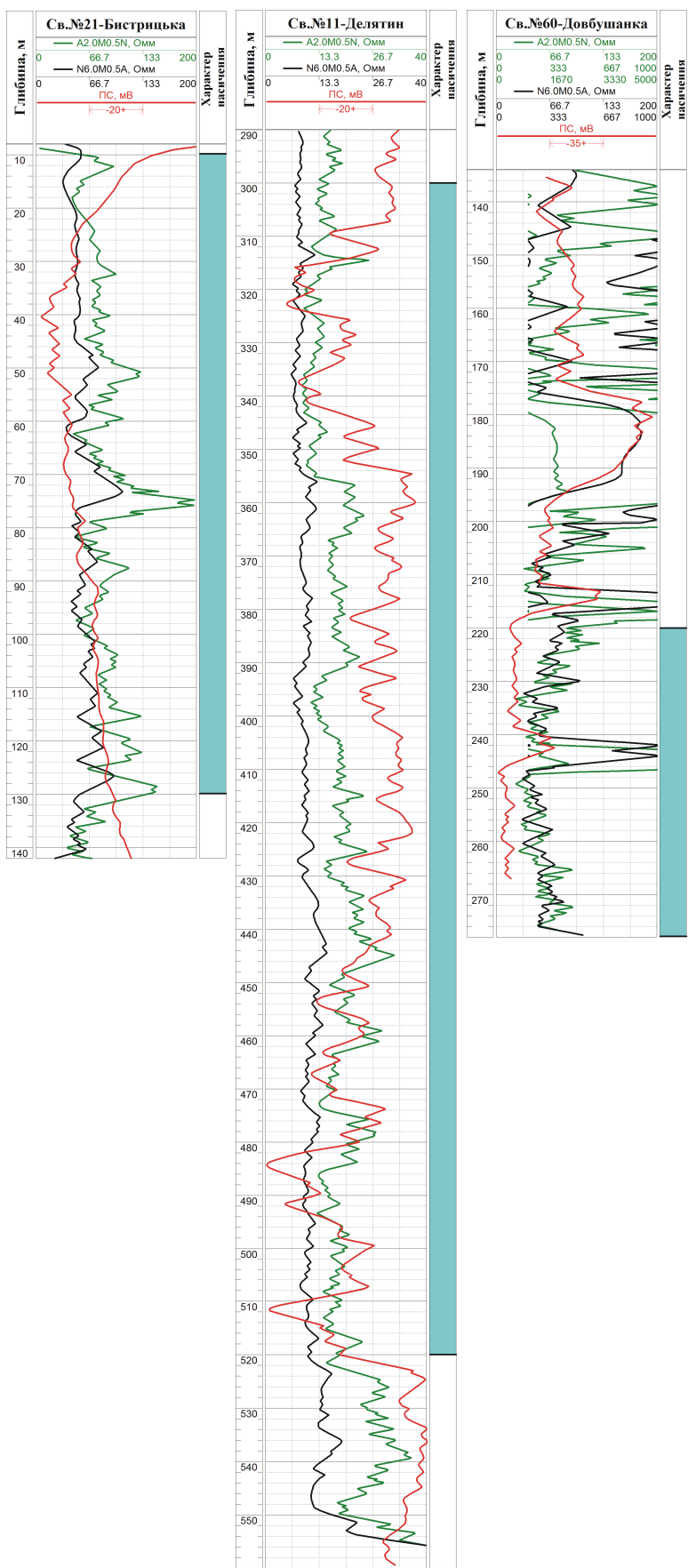
Рисунок 2 – Комплексна інтерпретація даних електрометрії при виділенні водоносних горизонтів у св. №21-Бистрицька, №11-Делятин, №60-Довбушанка
