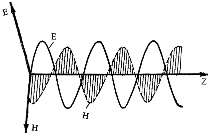
Рисунок 1 – Плоска електромагнітна хвиля в металевому ободі гальмівного шківів з його зовнішньої поверхні
