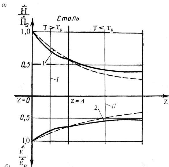
Рисунок 2 – Розподіл співвідношень напруженостей магнітного (а) та електричного (б) полів у сталі іззовні обоє шків при розв’язку приповерхневої (криві 1) та двошарової (криві 2) задачі за умов T > T_K та T < T_K
