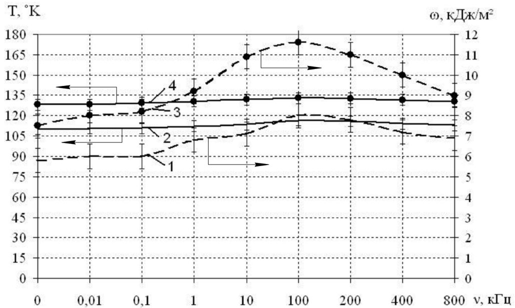
1 і 2 – криві залежності для епоксидної матриці; 3 і 4 – криві залежності для композиції з феритовим наповнювачем Штриховою лінією позначені криві параметрів ударної в'язкості, суцільною лінією позначені криві параметрів теплостійкості
