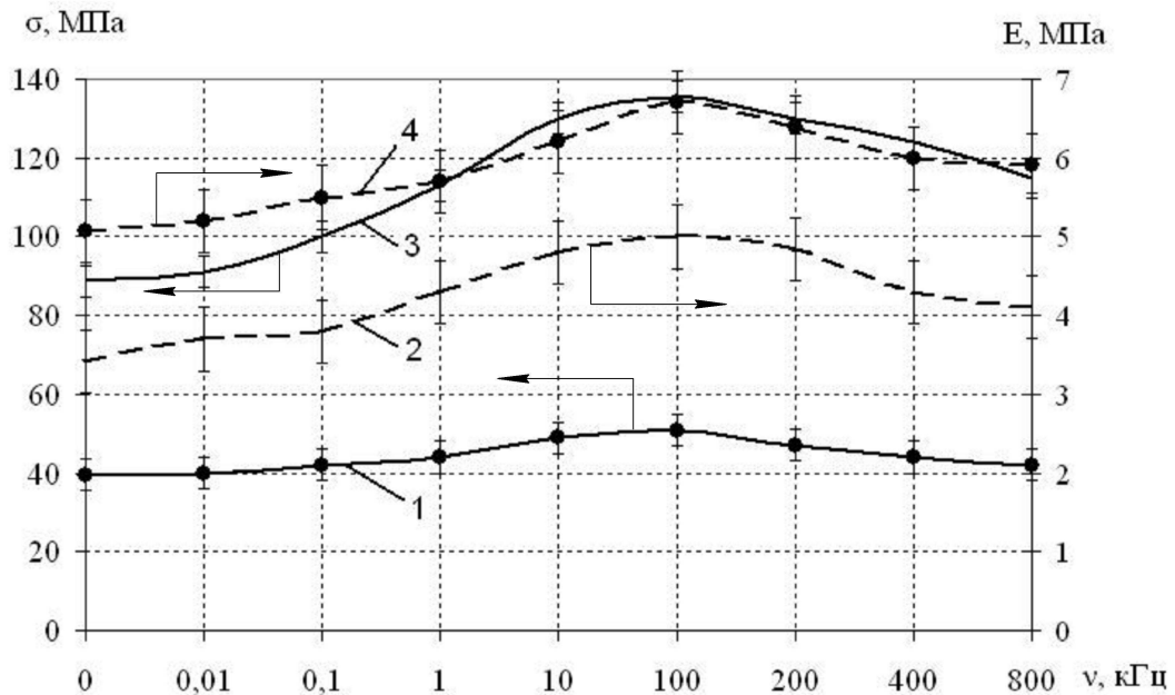
1 і 4 – криві залежності для епоксидної матриці 2 і 3 – криві залежності для композиції з феритовим наповнювачем Штриховою лінією позначені криві параметрів модуля пружності, суцільною лінією позначені криві параметрів руйнівного напруження при згині
