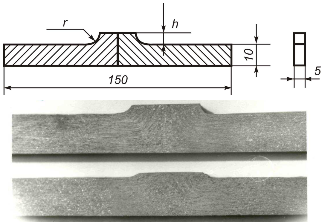
Рисунок 1 – Конструкція зразка для дослідження на опір втоми з контролем росту тріщин та поперечний шліф зварного з'єднання
