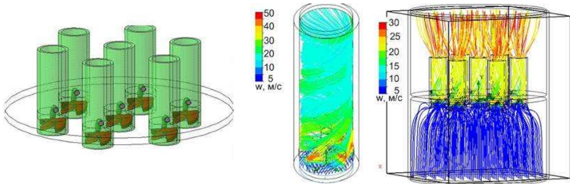
Рисунок 5 – 3D-модель тарілки з контактними елементами та траскторії руху газового потоку із заливками за значенням локальних швидкостей
