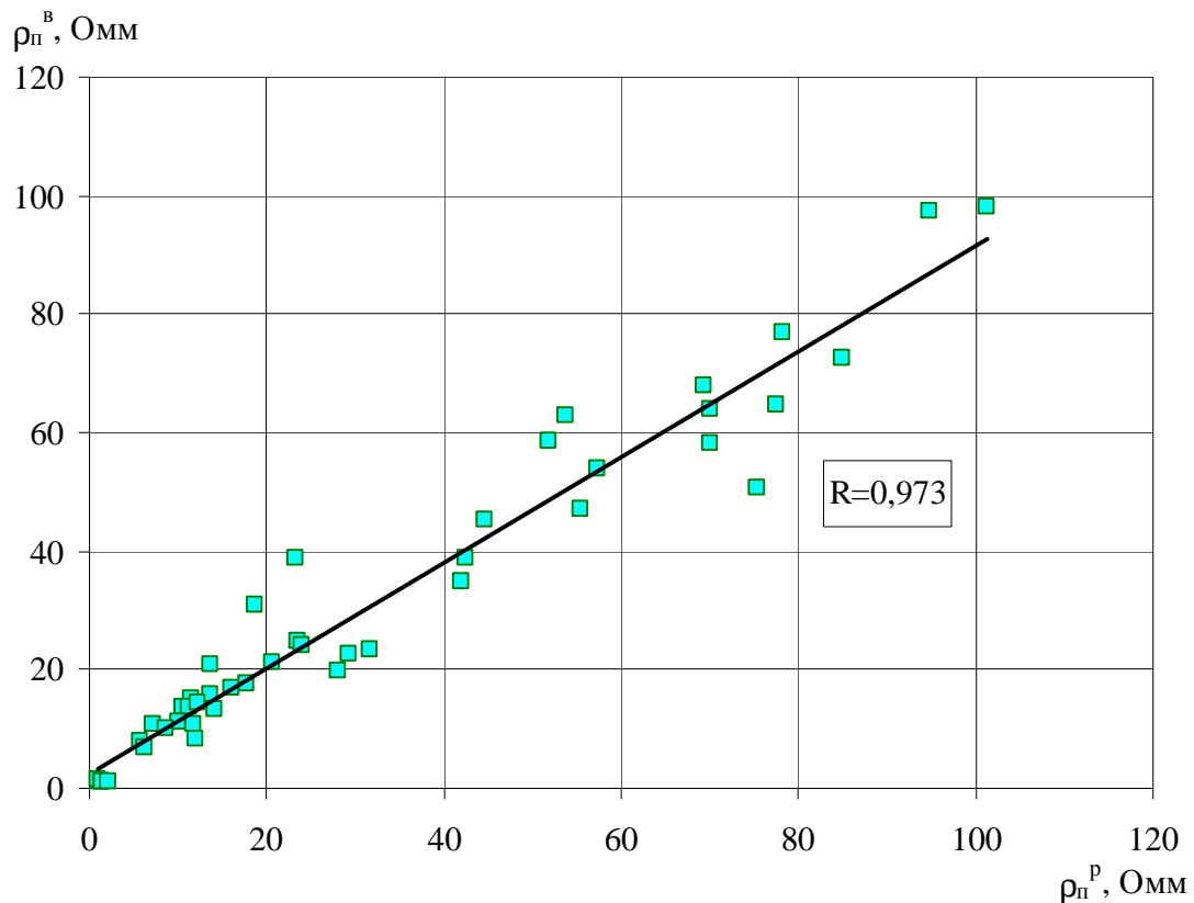
Рисунок 2 – Зіставлення питомого електричного опору \rho_n^B , виміряного на взірцях керну в лабораторних умовах, із розрахованими значеннями \rho_n^P (із врахуванням градієнта функції псевдокапілярметрії)
