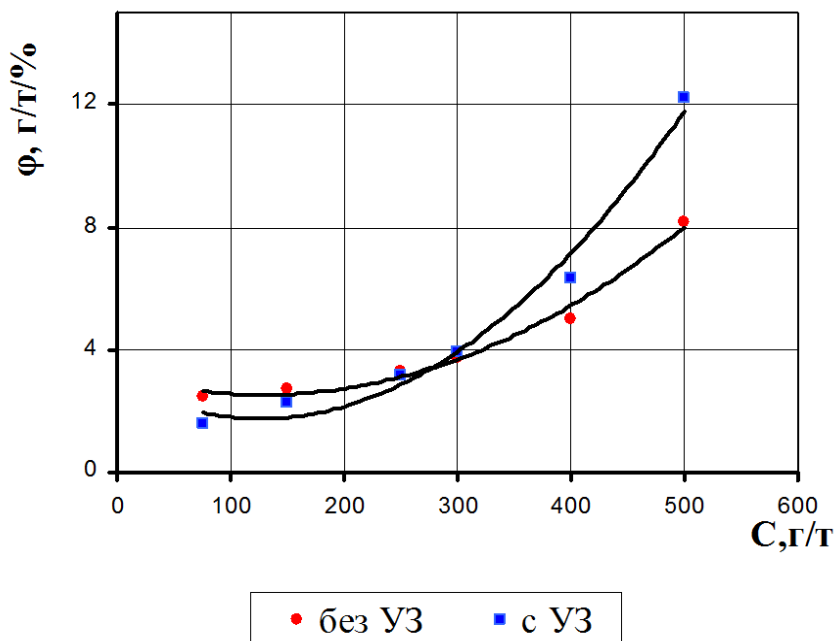
Рисунок 1 – Зависимость параметра удельной эффективности процесса деэмульсации от расхода реагента
