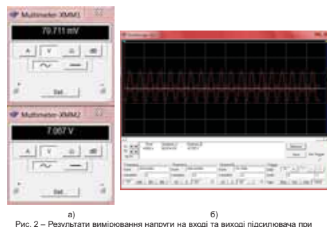
Рис. 2 – Результати вимірювання напруги на вході та виході підсилювача при частоті 100 Гц та синусоїдальній формі вхідного сигналу в середовищі Electronics Workbench
