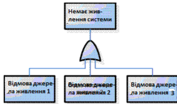
Рисунок 3 – Приклад застосування логічного знака «два з трьох»
