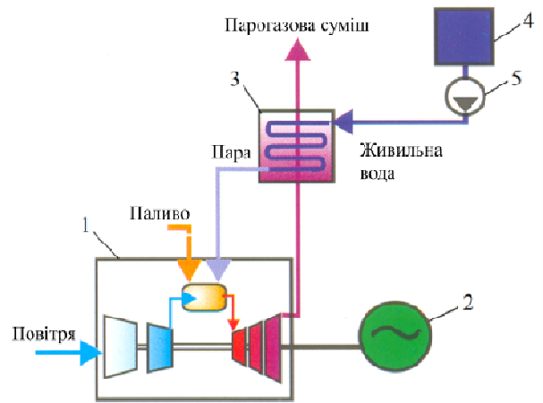
1 - ВМД; 2 - генератор; 3 - котел-утилізатор, 4 - РПВ; 5-насос
