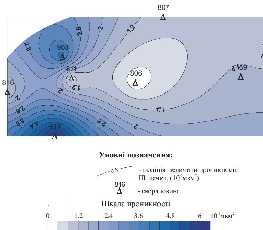
Рисунок 3 – Схема проникності ІІІ продуктивної пачки Пасічнянського нафтового родовища
