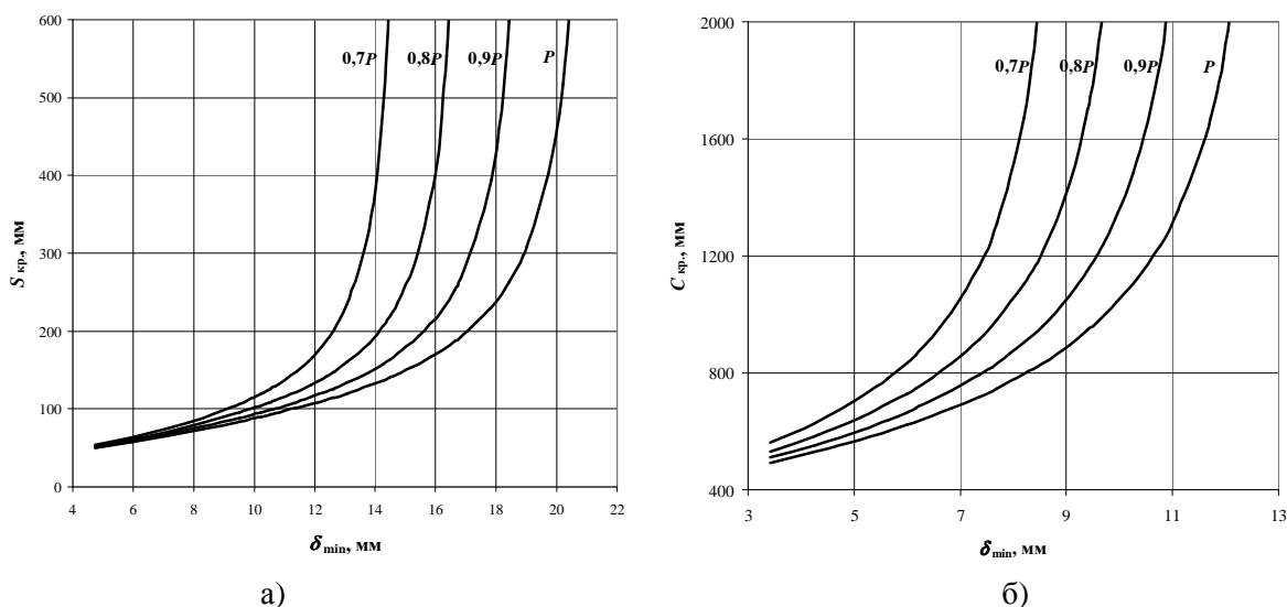
а) S_{ср.} ; б) C_{ср.} . Рисунок 2 – Диаграмма критических линейных размеров утонений стенки трубы из стали X70 диаметром 1420 мм
