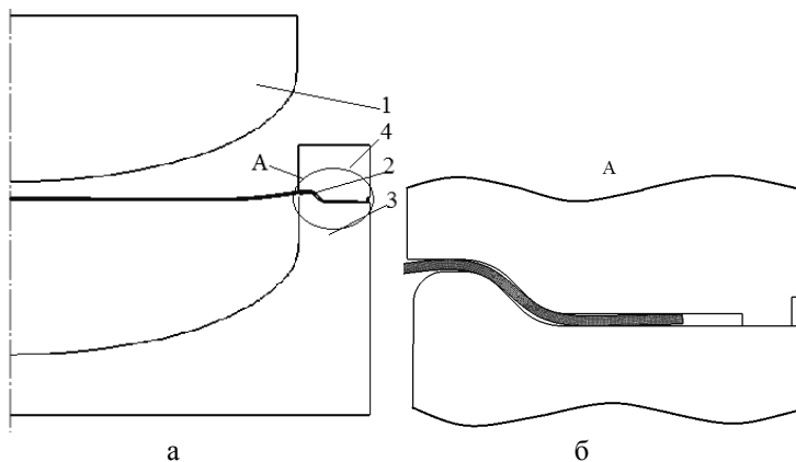
Рис. 1. Схема вытяжки заготовки (1 - пуансон; 2 - заготовка; 3 - матрица; 4 - прижимное кольцо)
