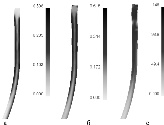
Рис. 2. Распределение напряжений и деформаций во фланце заготовки на конечной стадии вытяжки: а – логарифмической деформации; б – интенсивность деформации; с – интенсивность напряжений
