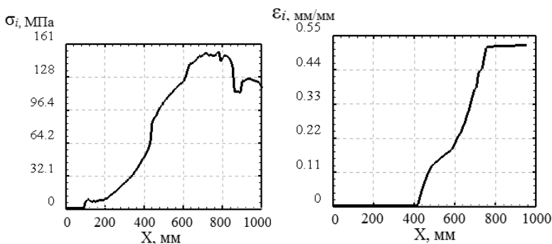
Рис. 4. Зависимость: а – интенсивность напряжения \sigma_i от перемещения пуансона X; б - интенсивность деформации \varepsilon_i от перемещения пуансона X
