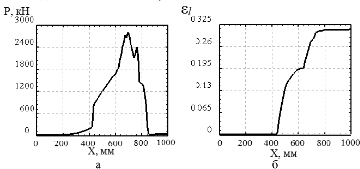
Рис. 3. Зависимость: а - силы вытяжки P от перемещения пуансона X ; б - логарифмической деформации \varepsilon_l от перемещения пуансона X
