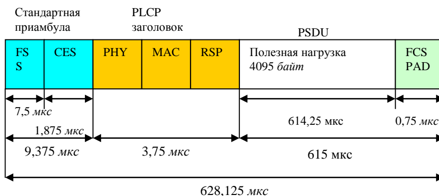
Рис. 2. Структура временных интервалов кадра для 53,3 Мбит/с
