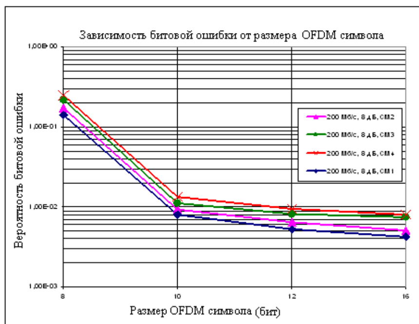
Рис. 10. Зависимость вероятности битовой ошибки от размера OFDM символа в битах
