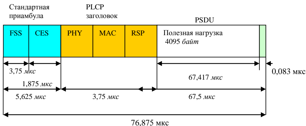
Рис.1. Структура временных интервалов кадра для 480 Мбит/с
