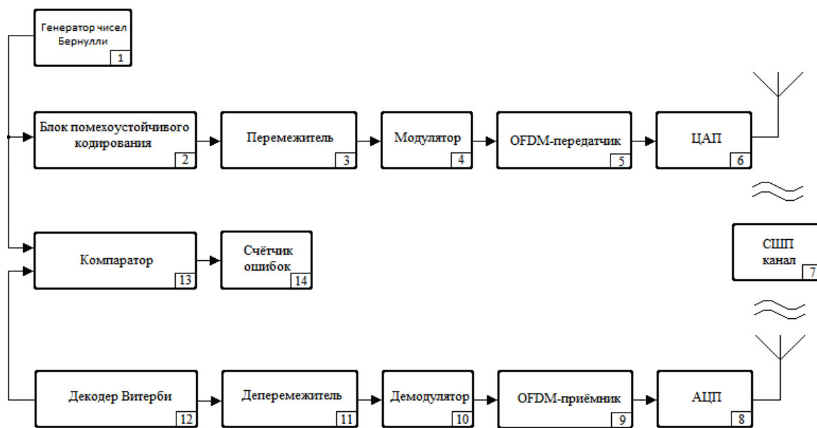
Рис. 4. Блок-схема модели СШП физического уровня
