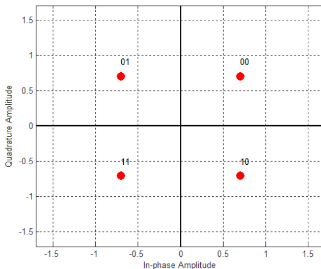
Рис. 6. Сигнальное созвездие QPSK
