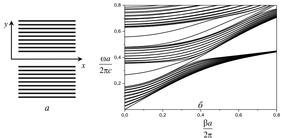
Рис. 1. Схема брэгговского пустотелого волновода и его дисперсионная
