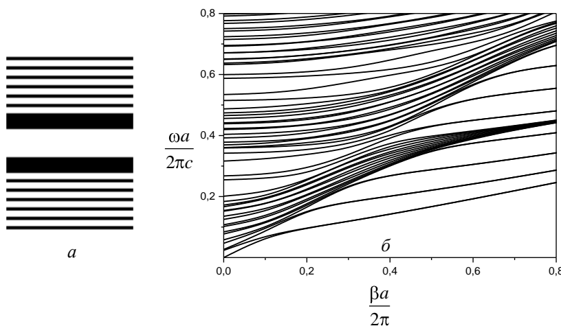
Рис. 2. Диэлектрический волновод с брэгговскими зеркалами
