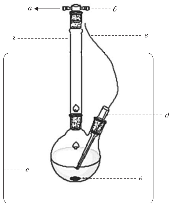
Рис. 2. Принципова схема установки для синтезу Флокаліну: a — відведення газоподібних продуктів; b — отвір для вирівнювання тиску; v — оптоволоконний датчик температури; z — повітряний холодильник; d — капіляр для датчика температури; e — корпус мікрохвильової системи «Mars»; e — магнітний перемішувач
