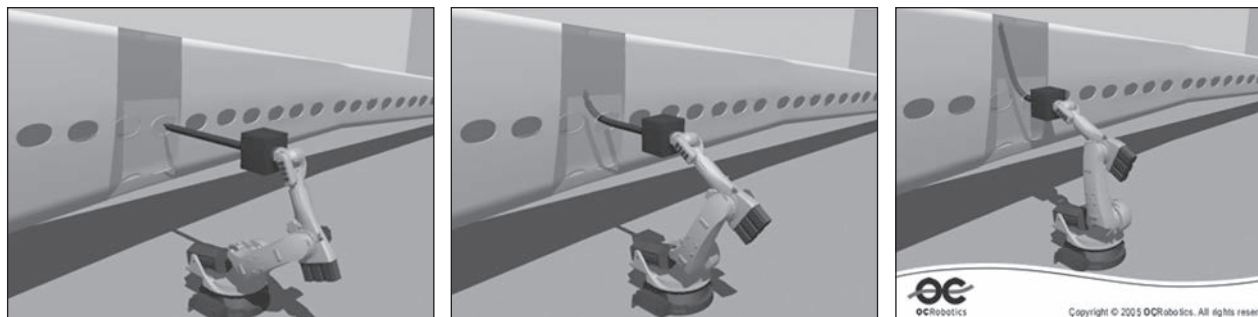
Рис. 2. Выполнение операций в кессоне крыла
