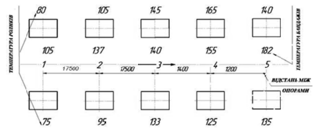
Рис. 2. Схема вимірювань температур на опорі
