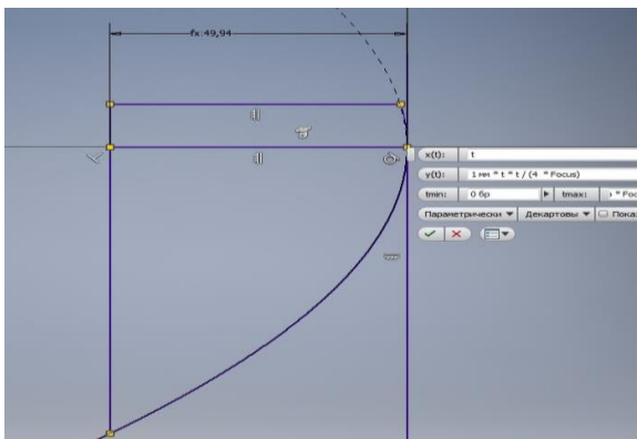
Побудова параболи обертання на базовому ескізі за формулою: y = \frac{x^2}{4 \cdot F} , де F - фокусна відстань
