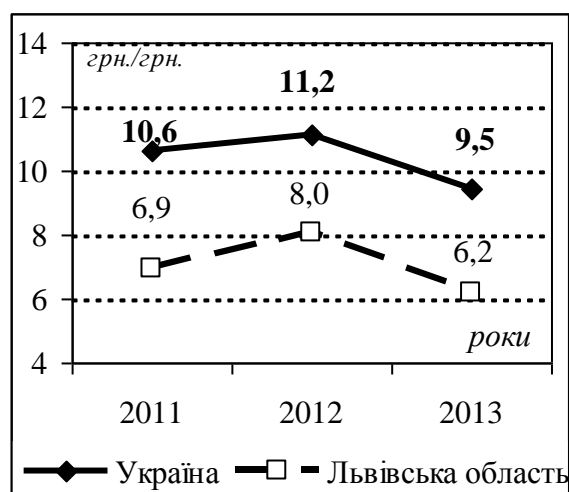
б) зарплатовіддача
