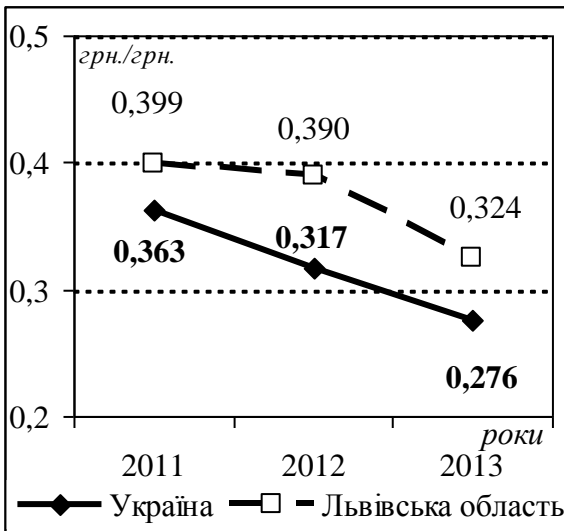
а) фондівіддача
