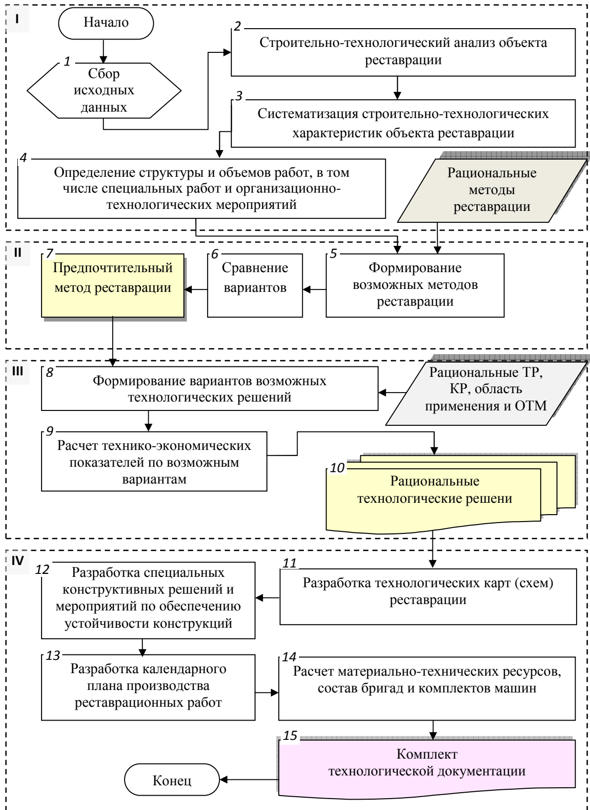
Рис. 1. Схема методики выбора рациональной технологии реставрации памятников архитектуры
