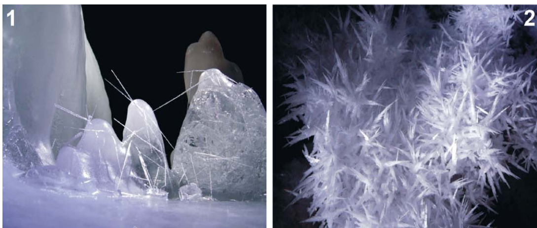
Рис. 8. Игольчатые (1) и перьевидные (2) сублимационные кристаллы. Fig. 8. Needle (1) and feather-shape (2) sublimation crystals.
