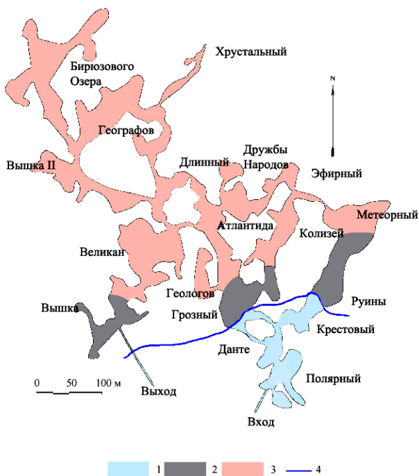
Рис. 2. Микроклиматические зоны Кунгурской Ледяной пещеры: 1 – зона постоянных отрицательных температур, 2 – переходная зона, 3 – нейтральная зона с практически постоянными температурами, 4 – граница распространения многолетнего оледенения.
