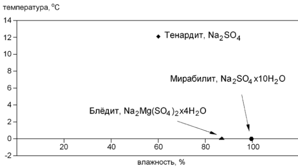
Рис. 39. Зависимость образования эфемерных минералов от температуры и влажности пещерного воздуха (поровых растворов). Fig. 39. Dependence of formation of ephemeral minerals from the temperature and humidity of the cave air (pore solutions).
