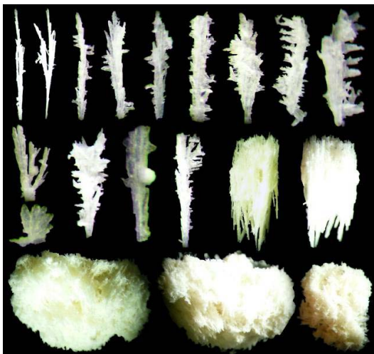
Рис. 17. Скелетные агрегаты гипса и фрагменты кристаллических корок, сложенных гипсом. Грот Скандинавский. Fig. 17. Skeletal gypsum aggregates and fragments of loose crystalline crusts composed from gypsum. The Scandinavian Grotto.
