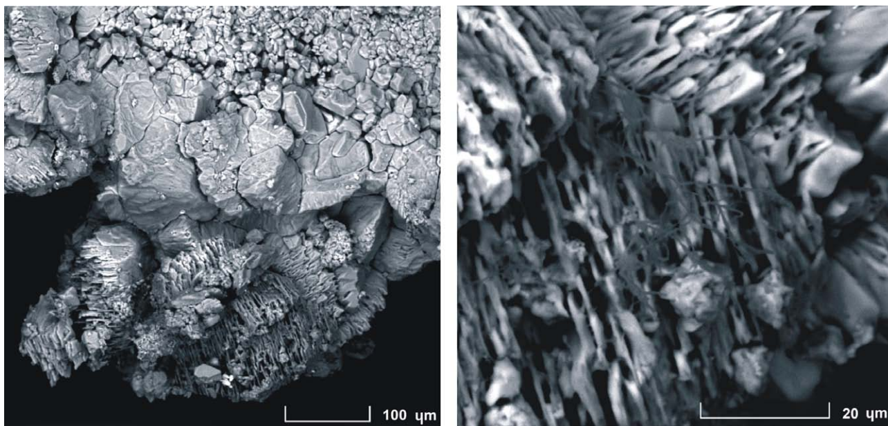
Рис. 25. Фрагмент поверхности гипсовой стенки в гроте Смелых под микроскопом: слева – элементы зональности (сверху вниз: первичный гипс, перекристаллизованный, корродированный), справа – грибной мицелий (?) на фоне корродированной поверхности.
