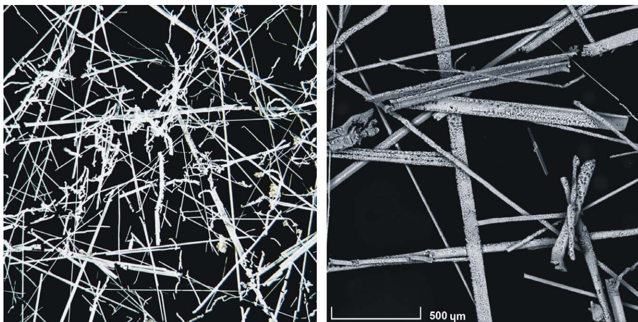
Рис. 23. Игольчатые кристаллы мирабилита, сформировавшиеся на полиминеральной подложке.
