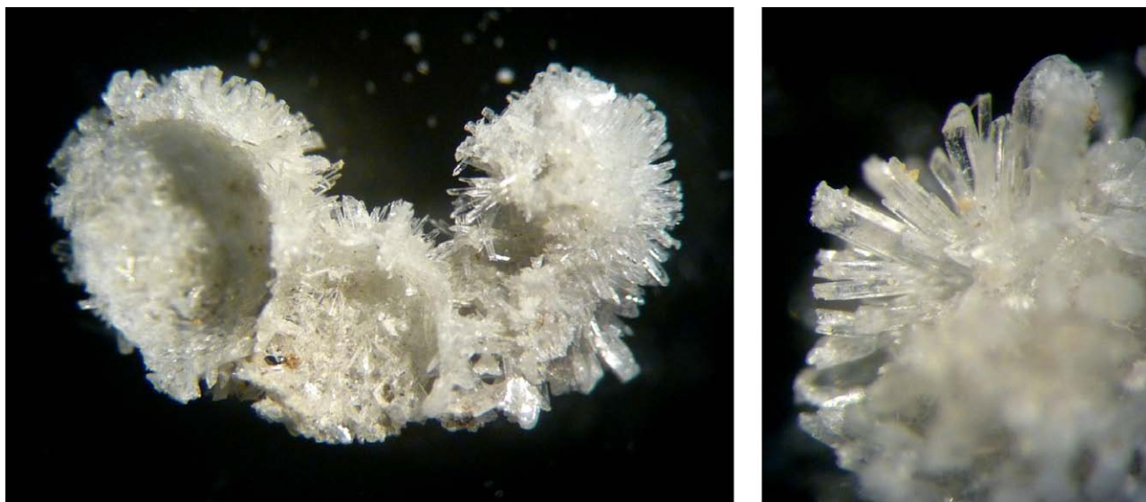
Рис. 15. Вид внутренней части гипсовых кристаллов и справа – вид отдельных крупных кристаллов (грот Скандинавский). Fig. 15. Kind of internal gypsum crystals and on the right – a kind of separate large crystals (Scandinavian Grotto).
