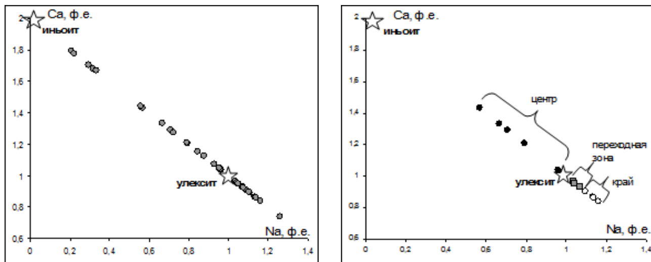
Рис. 22. Вариации состава боратов из грота Смелых (левый график), в том числе – в пределах отдельных зональных конкреций (правый график)
