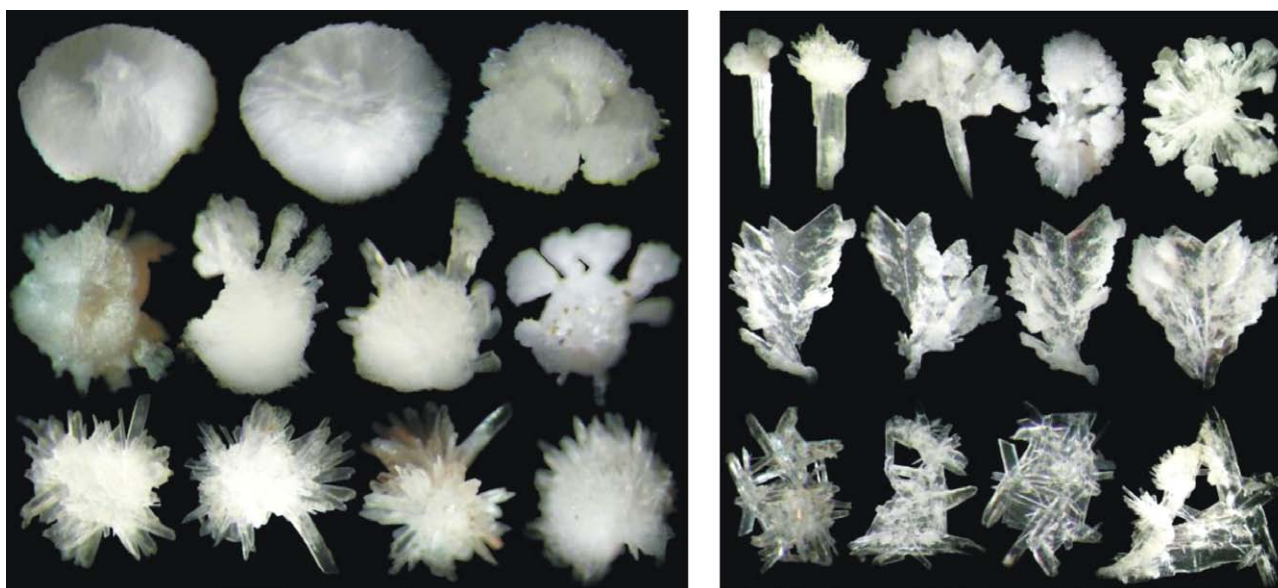
Рис. 16. Сферолиты, в различной степени регенерированные, иногда с признаками двух стадий расщепления (слева), расщепленные кристаллы гипса и плоские агрегаты (двойники и сростки - справа). Грот Скандинавский. Fig. 16. Spherulites, in varying degrees, recovered, sometimes with signs of the two stages of splitting (left), the splintered gypsum crystals and flat aggregates (twins and intergrowths – right). The Scandinavian Grotto.
