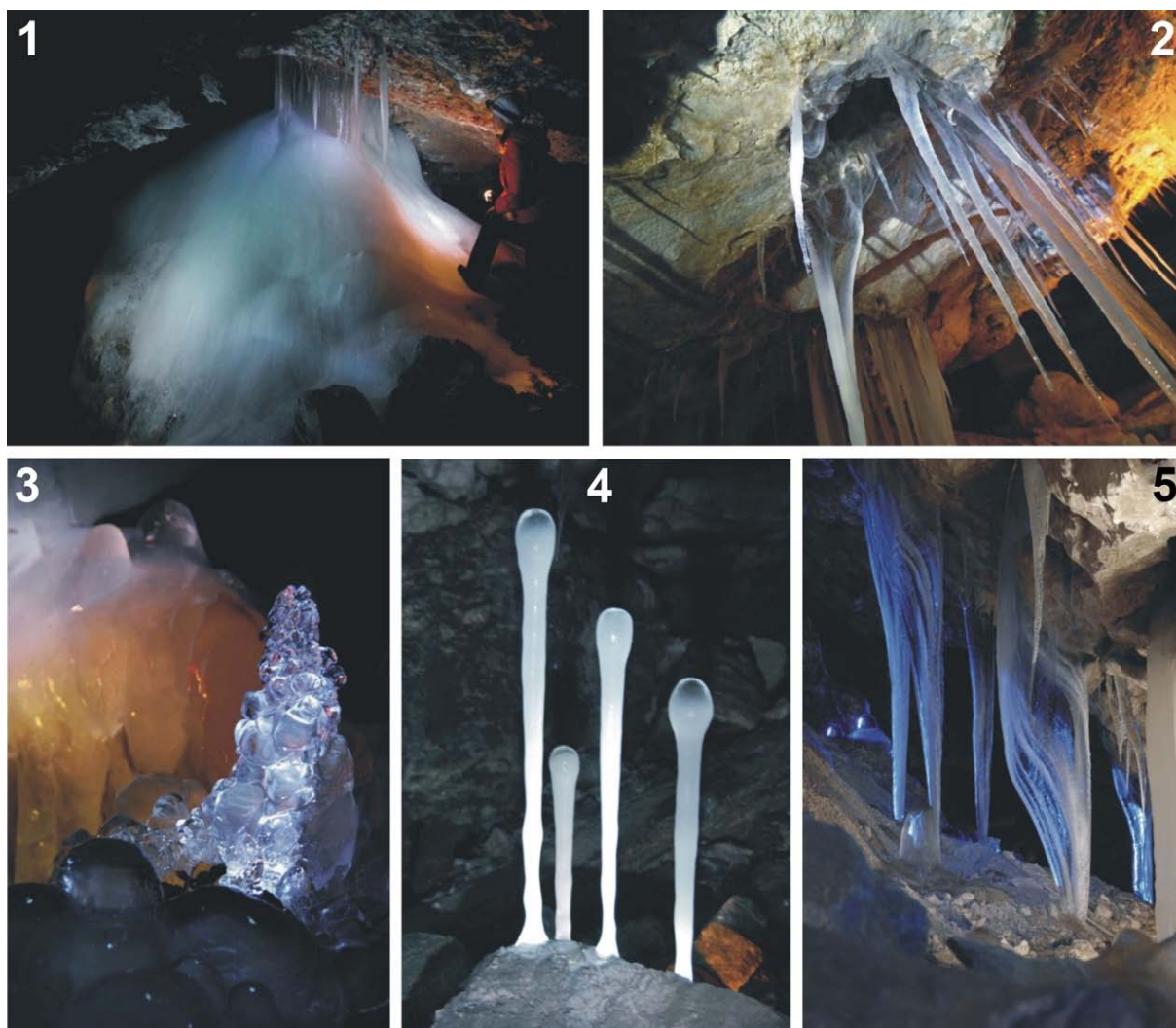
Рис. 4. Некоторые формы натечных конжеляционных льдов Кунгурской Ледяной пещеры: 1 – покровная наледь, 2 – сталактиты, 3 – «шаровые» сталагмиты, 4 - булавовидные сталагмиты, 5 – занавеси. Fig. 4. Some forms of ice sinters in Kungur Ice Cave: 1 – covering naled, 2 – stalactites, 3 – ball stalagmites, 4 – club-shaped (mace-shaped ?) stalagmites, 5 – draperies.
