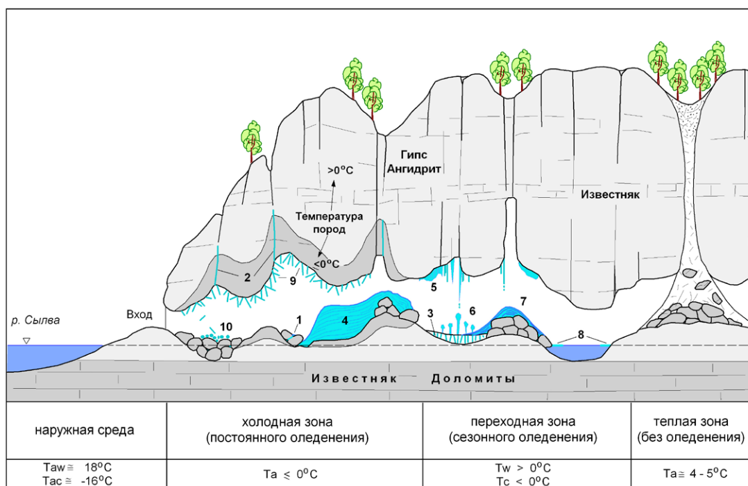
Рис. 3. Микроклиматические зоны Кунгурской Ледяной пещеры и характерные для них типы снежно-ледовых образований: 1–поровый лед, 2–жильный лед (в трещинах), 3 – сегрегационный лед, 4 – многолетний слоистый лед (наледь), 5 – висячие наледи (сталактиты, драпировки и т.д.), 6 – сталагмиты, 7 – покровная наледь, 8 – озерный лед, 9–сублимационный лед (пещерный иней).
