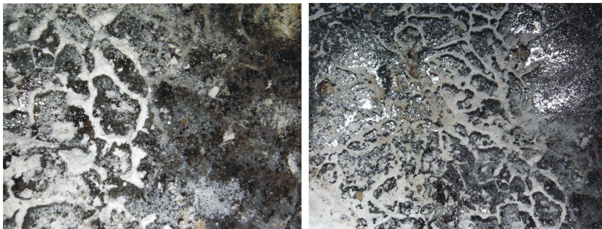
Рис. 11. Агрегирование гипсовой муки с образованием полигональных структур в результате механического обособления минеральных примесей по границам перекристаллизованных индивидов льда
