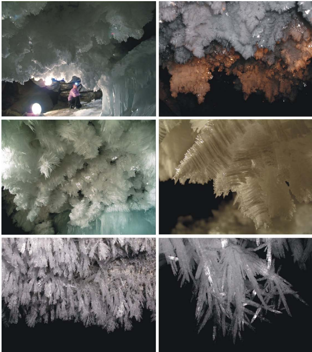
Рис. 7. Сублимационные кристаллы «пещерного инея» на сводах пещеры. Fig. 7. Sublimation crystals of «cave frost» on the arches of the Cave.
