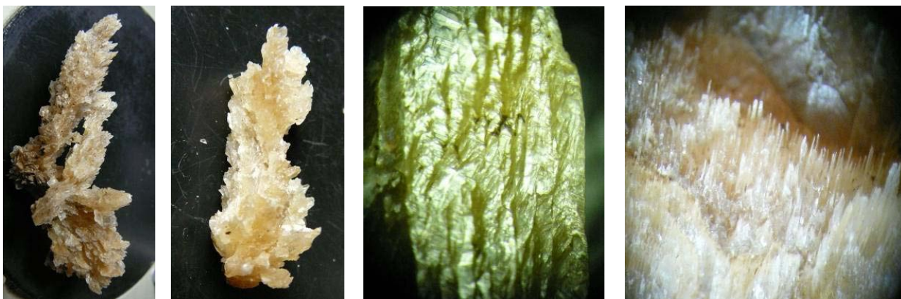
Рис. 31. Отдельные расщепленные индивиды гипса, выросшие в глине в гроте Грязный и детали их строения (блочность и игольчатая поверхность). Fig. 31. Split individual gypsum aggregates grew out of clay in the Dirty Grotto with details of their structure (blocking and needle surface).
