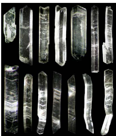
Рис. 30. Искривленные кристаллы гипса с полосами трансляционного скольжения. Грот Географов. Fig. 30. Curved gypsum crystals with strips of translational slip. The Geographer's Grotto.
