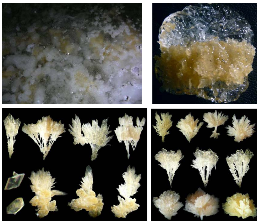
Рис. 13. Отдельные игольчато-скелетные дендриты, в различной степени регенерированные (слева), зональные агрегаты, отдельные кристаллы и наросты на них расщепленные индивиды. Грот Первый (проба № 2). Fig. 13. Sample N 2. Gypsum aggregates inside the ice mass body (top left), a sample (top right). Separate acicular-skeleton dendrites in different stages of regeneration (bottom left), zonal aggregates and separate crystals with split individuals formed on them (bottom right).
