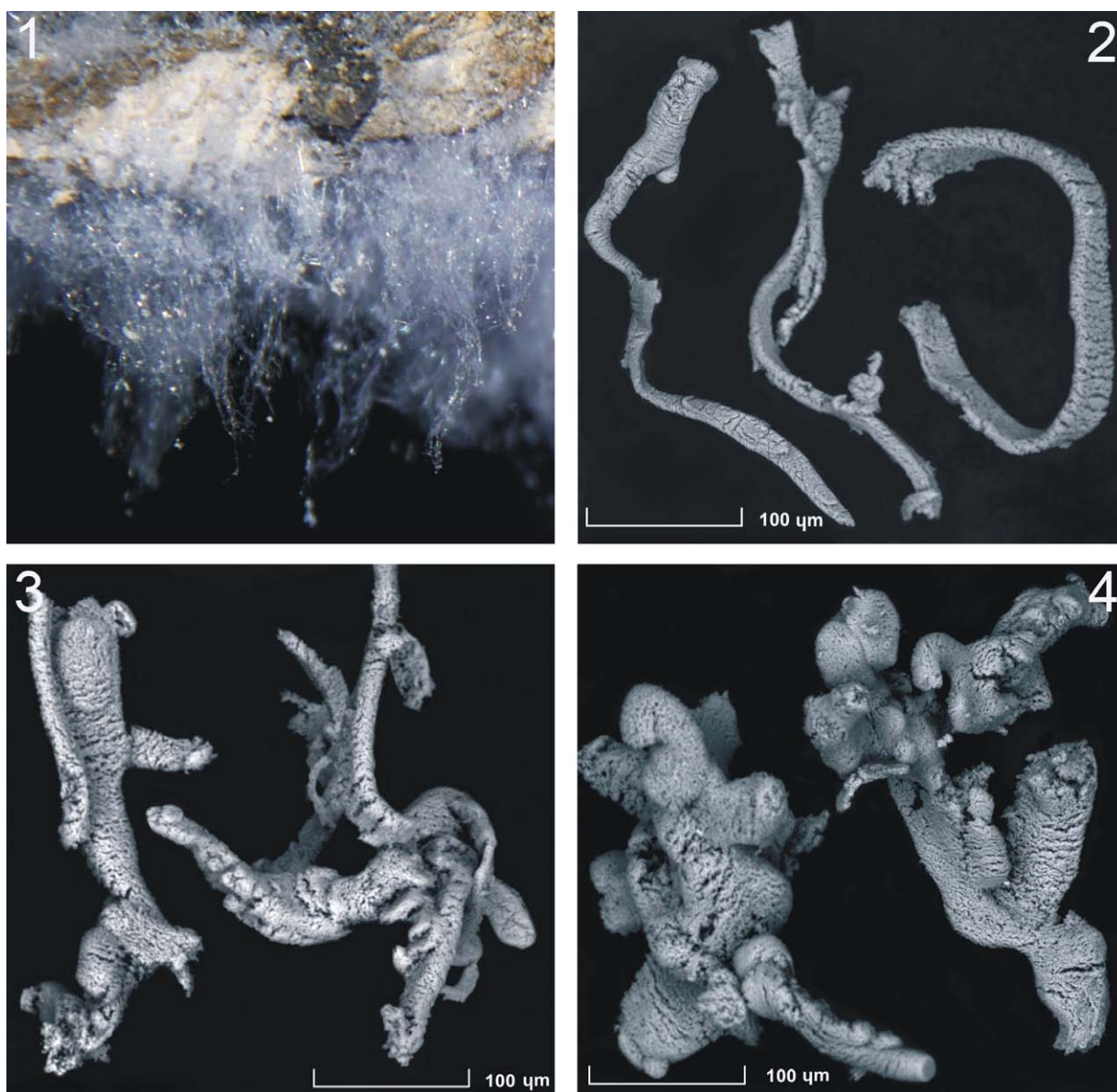
Рис. 24. Общие виды агрегатов и субиндивидов мирабилита, сформировавшихся на стенах: 1 – игольчатый агрегат, растущий с подложки в естественных условиях, 2-4 – субиндивиды мирабилита под микроскопом.
