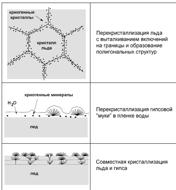
Рис. 37. Различные случаи эпигенетической трансформации льда и криогенной минерализации. Fig. 37. Various cases of epigenetic transformation of ice and cryogenic minerals.
