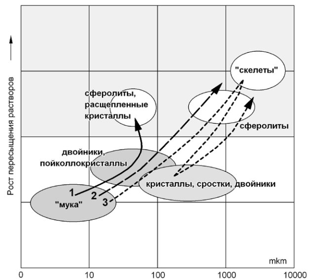
Рис. 38. Модель эволюции криогенных образований гипса в Кунгурской пещере. Тренды: 1 – вымораживания (собственно криогенный); 2 – перекристаллизации увлажненной муки; 3 – перекристаллизации как льда так и гипсового материала в условиях многолетних температурных колебаний. Fig. 38. Model of evolution of cryogenic gypsum formations in Kungur Ice Cave. Trends: 1 – freezing (actually cryogenic) 2 – recrystallization of moistened flour, 3 – recrystallization of both ice and gypsum material of flour in temperature fluctuation conditions.
