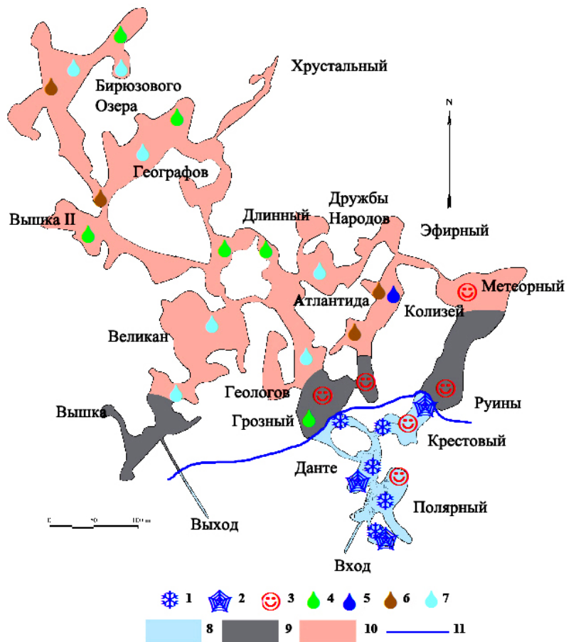
Рис. 40. Распределение современных минеральных образований в Кунгурской Ледяной пещере: 1 – криогенных; 2 – криогенно-перекристаллизованных; 3 – экструзивных; 4-7 – кристаллизующихся из водных растворов (4 – в ванночках, 5 – из стекающей пленки, 6 – в глинистом субстрате, 7 – за счет аэрации водных растворов). Микроклиматические зоны: 8 – зона постоянных отрицательных температур, 9 – переходная зона, 10 – нейтральная зона с практически постоянными температурами, 11 – граница многолетнего оледенения.
