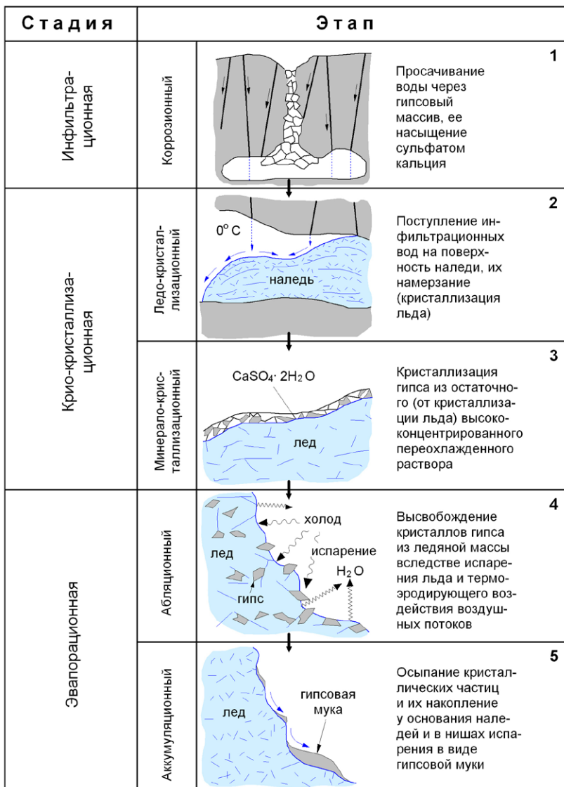
Рис. 35. Схема формирования криоминеральных мучнистых отложений у подножья подземных наледей в Кунгурской Ледяной пещере (Андрейчук, Галускин, 2001; рисунки, отражающие стадии, разномасштабны). Fig. 35. Scheme of cryomineral mealy sediments formation at the foot of cave nales in Kungur Ice Cave (Andreychouk, Galuskin, 2001; figures reflecting the stages are given in different scale).
