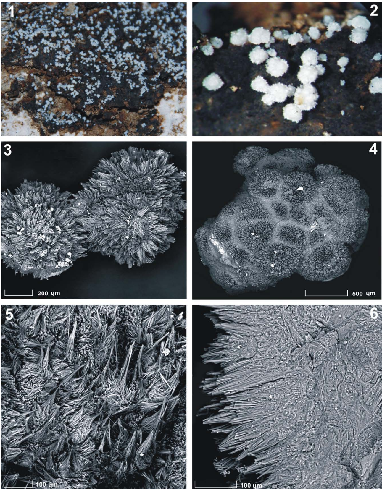
Рис. 21. Морфология выделений улексита: 1 – общий вид улекситовой «россыпи», 2 – увеличение рис. 1, 3 – моноцентрические конкреции, 4 – полицентрическая конкреция, 5 – элементы нижней поверхности, 6 – характер внутреннего строения.
