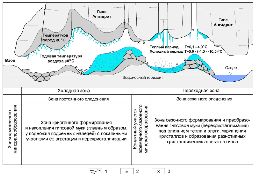
Рис. 9. Приуроченность криоминеральных образований к разным микроклиматическим зонам пещеры: 1 – гипсовая мука, 2 – криоминеральные агрегаты, формирующиеся путем перекристаллизации гипсовой муки, 3 – участки с эфемерными криоминеральными образованиями.
