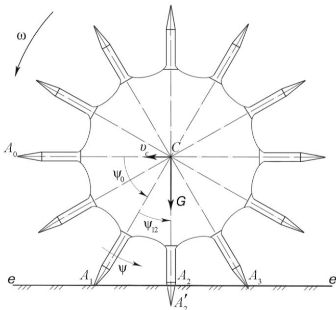
Рис. 1 – Схема диска борони з іглами при його русі вліво і повороті
