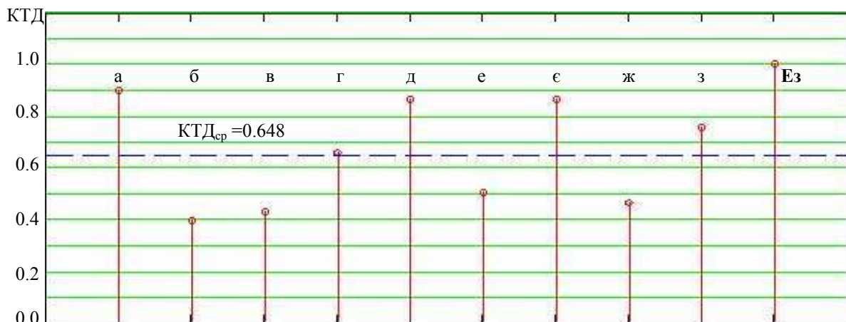
Рис. 2 Гістограма залежності КТД обраних зразків-аналогів а- Argus-M2; б- «Радіан-02»; в- «Охота»; г- МКТК-1А; д- Леер-2; е- «Барс-ВЧ»; є- «Лорандит-М»; ж- «Свет-КУ»; з- CRS-8000; Ез – Еталонний зразок
