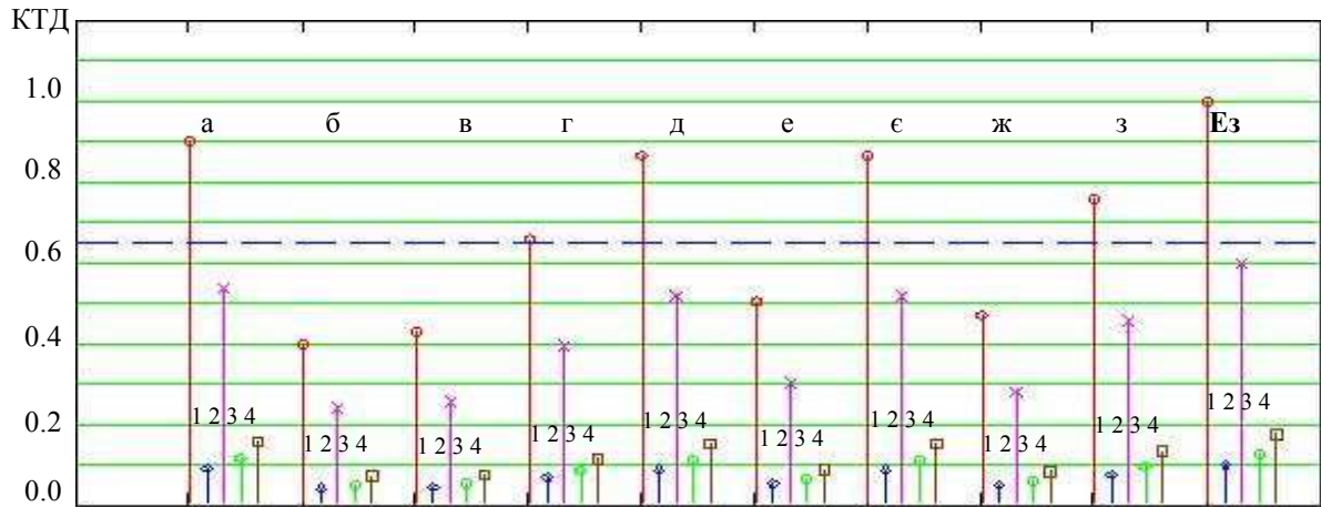
Рис. 3 Коефіцієнти технічної досконалості зразків-аналогів з деталізацією їх складових за групами декомпозиції а- Argus-M2; б- «Радіан-02»; в- «Охота»; г- МКТК-1А; д- Леер-2; е- «Барс-ВЧ»; е- «Лорандит-М»; ж- «Свет-КУ»; з- CRS-8000; з- Еталонний зразок
