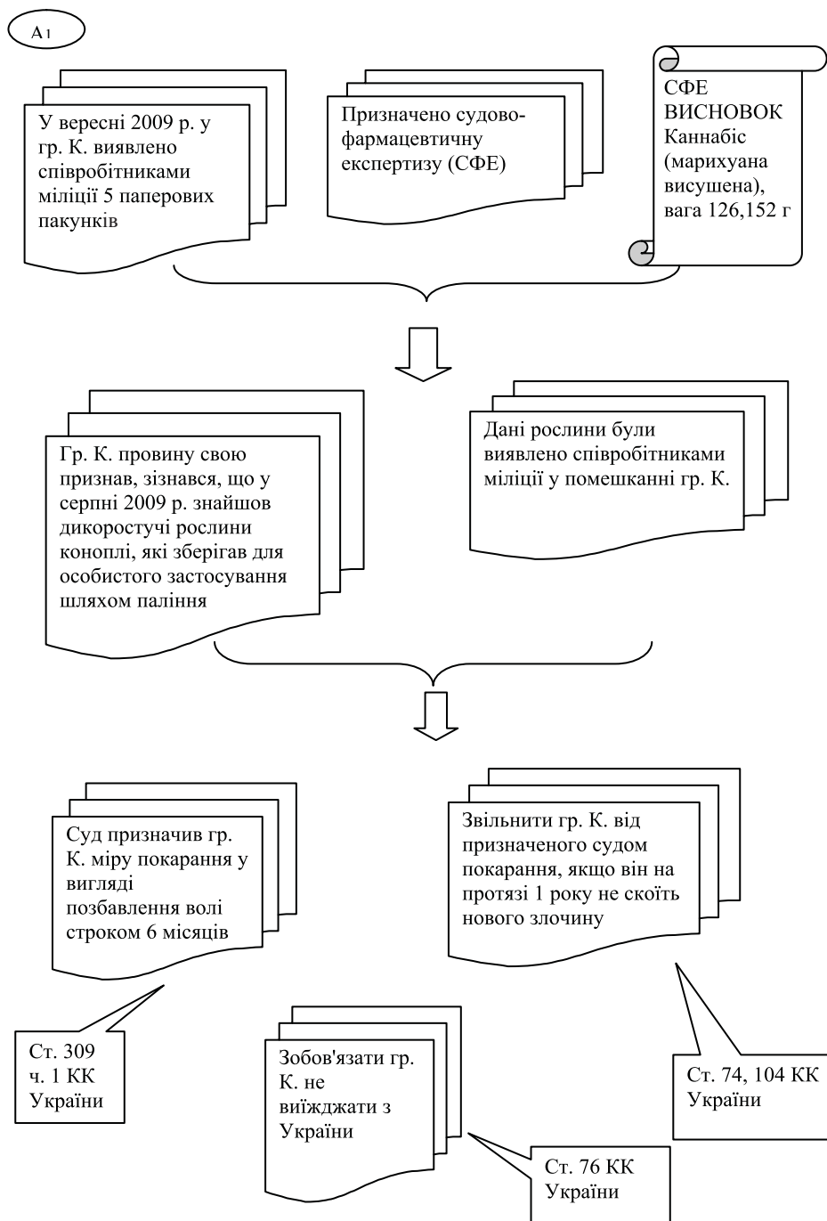
Мал. 1 Схематичне зображення подій із судово-фармацевтичного прикладу
