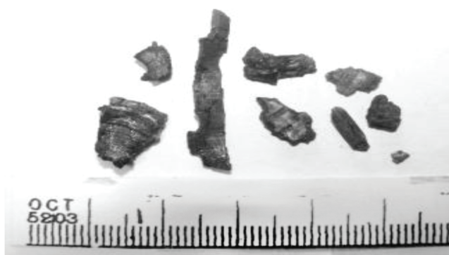
Рис №9. Уламки від корпусу ВОГ-17М
