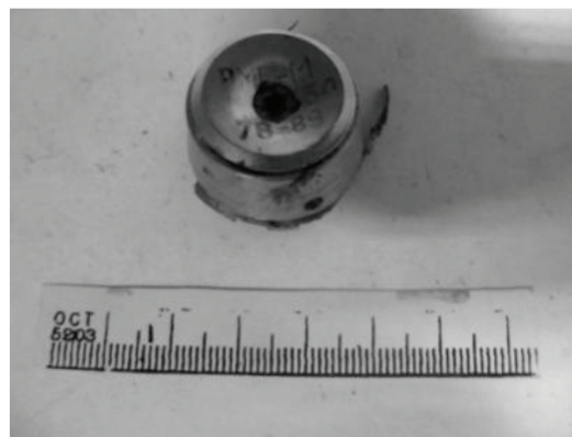
Рис №8. Фрагмент головного підричника ВОГ-17М зі збереженням маркуванням
