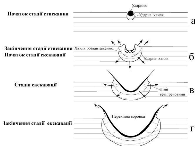
Рис. 5. Діаграми, які схематично у розрізі показують утворення ударних кратерів в багат шаровій мішені:
