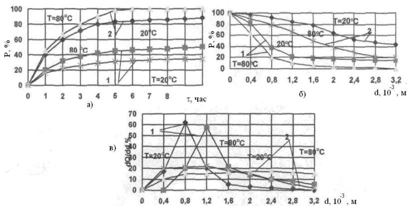
Рис.2.: а - седиментационное накопление; б - кумулятивные кривые накопления; в - интегральные кривые распределения размеров каплей: 1 - граничной и 2 - крупной фракций.
