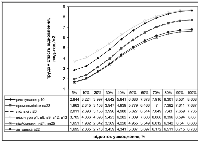
Рис. 2. Залежність середньої трудомісткості відновлювальних робіт із застосуванням різних засобів підмоцвання від площі ушкодженої теплоізоляції розглянутих в обчислювальному експерименті будівель-представників
