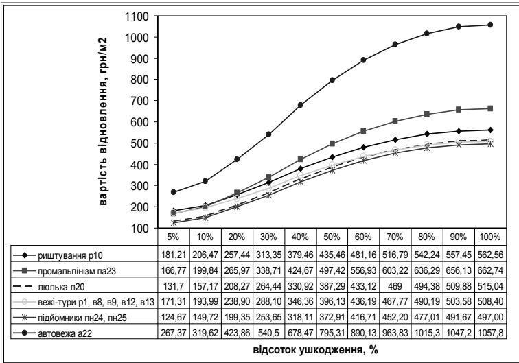
Рис. 1. Залежність середньої вартості відновлювальних робіт із застосуванням різних засобів підмоцнення від площі uszkodженої теплоізоляції розглянутих в обчислювальному експерименті будівель-представників
