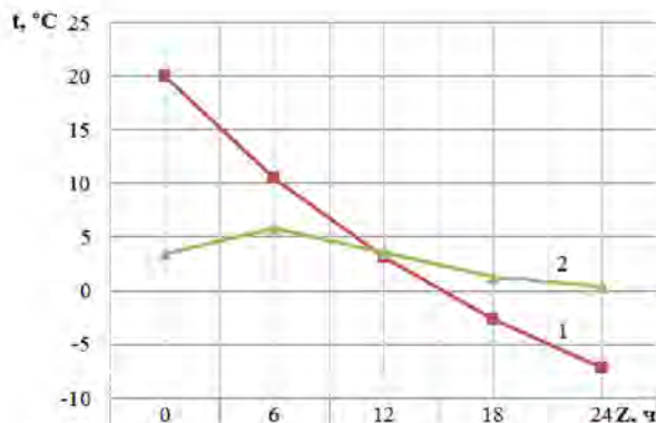
Рис. 1. Изменение температуры внутреннего воздуха помещения и градиента температур ( t_{в} - t_{г} ) при охлаждении из стационарного состояния для 1 типа здания при вводе в эксплуатацию ( P = 800 \text{ кДж/м}^3 )
