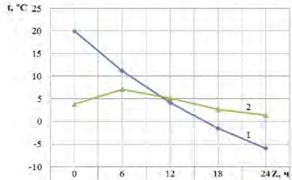
Рис. 2. Изменение температуры внутреннего воздуха помещения и градиента температур ( t_{в} - t_{г} ) при охлаждении из стационарного состояния для 1 типа здания при длительной эксплуатации ( P = 864 \text{ кДж/м}^3 )
