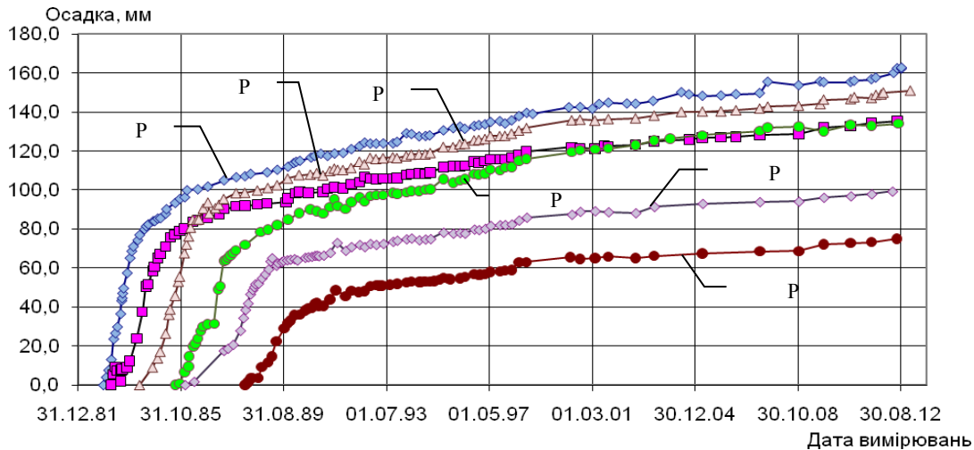
Рис. 1. Графіки розвитку осідань будівель РВ-1...6 Запорізької АЕС / Graphs of building subsidence РВ-1 ... 6 Zaporizhia nuclear power plant
