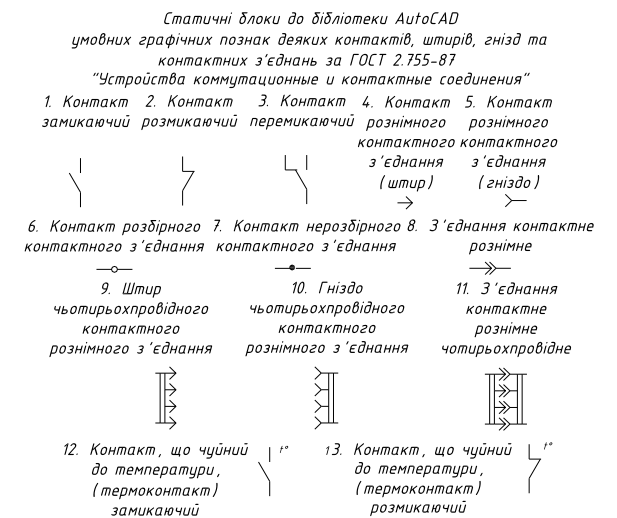
Рис. 6. Файл “Пристрої комутаційні і контактні з'єднання за ГОСТ 2.755-87 (сблоки).dwg” / File “Switching device and contact connections State Standard (static blocks).dwg”
