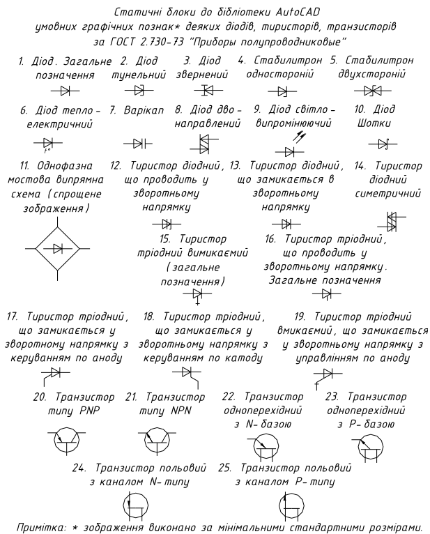
Рис. 3. Файл “Напівпровідникові елементи за ГОСТ 2.730-73 (сблоки).dwg” / File “Semiconductors State Standard 2.730-73 (static blocks).dwg”
