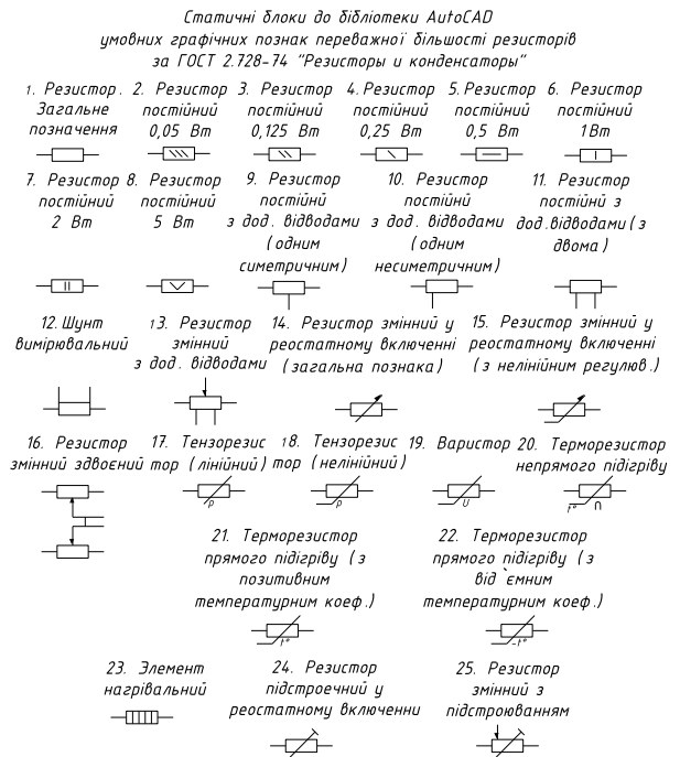
Рис. 5. Файл “Резистори за ГОСТ 2.728-74 (сблоки).dwg” / File “Resistors State Standard 2.728-74 (static blocks).dwg”
