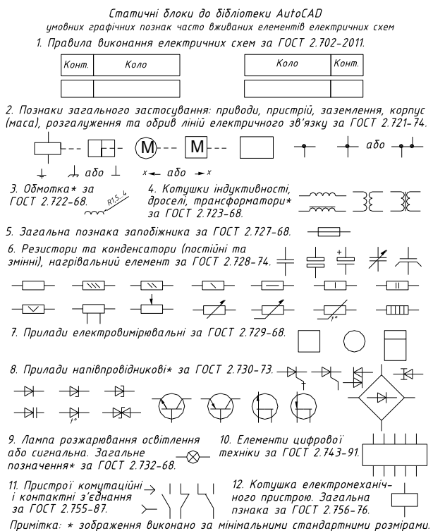
Рис. 4. Файл “Позначки деяких часто вживаних елементів (сблоки).dwg” / File “Some refer to frequently used items (static blocks).dwg”
