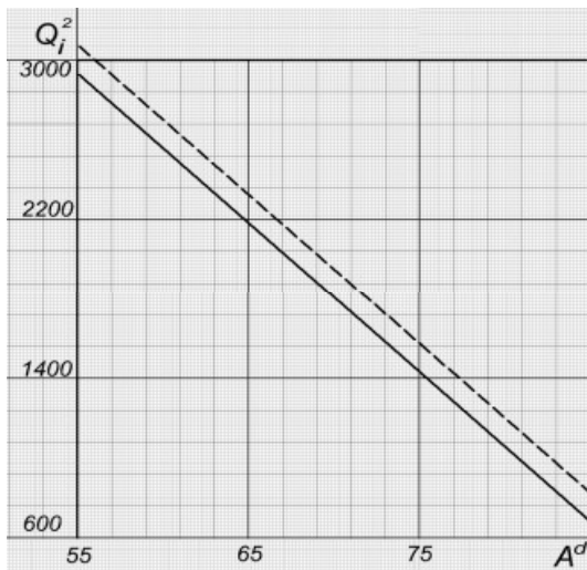
Рис. 1 Графическая зависимость нижней теплоты сгорания рабочего топлива в отходах углеобогащения (влажностью 8,9 %) от зольности / Graphical dependence of lower operating heat of combustion of the waste coal preparation (humidity 8.9%) from the ash.
