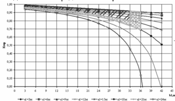
Рис. 2 Показатель безопасной организации зоны производства работ (при схемах организации зоны производства работ № 3) / Index of safe organization of execution area production of works (schemes of the organization of the area production of works № 3)
