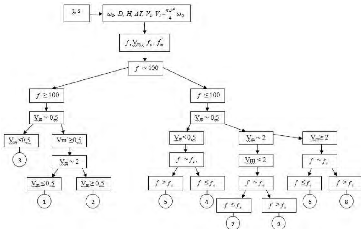
Рис.1. Блок-схема определения максимальных приземных концентраций C_m / Flowchart of determination of the maximum ground concentration C_m
