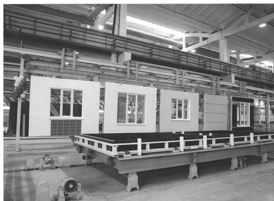
Рис.4. Примеры декоративной отделки стеновых панелей / Examples of the decorative finishing of a wall panel
