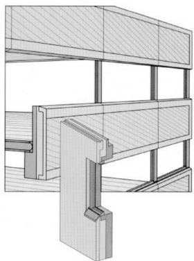
Рис.2. Схематическая конструкция стеновой панели / Schematic construction of a wall panel
