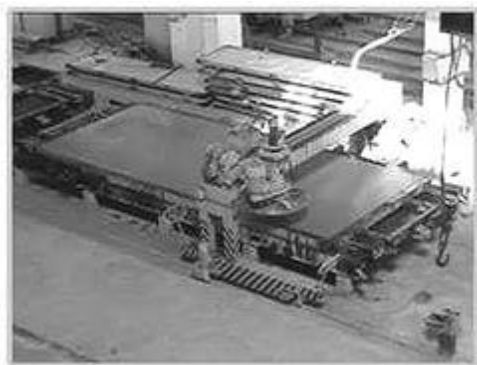
Рис.6. Производство стеновой панели в стационарном поддоне / A production of a wall panel is in a stationary pallet
