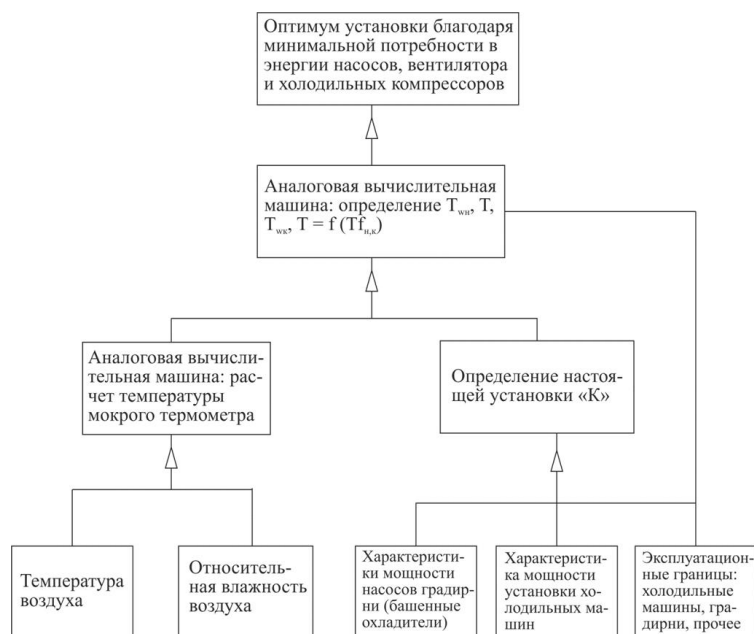
Рис. 2 Способ действия системы регулирования работы холодильной установки / Method of operation of the system control the operation of the refrigeration unit
