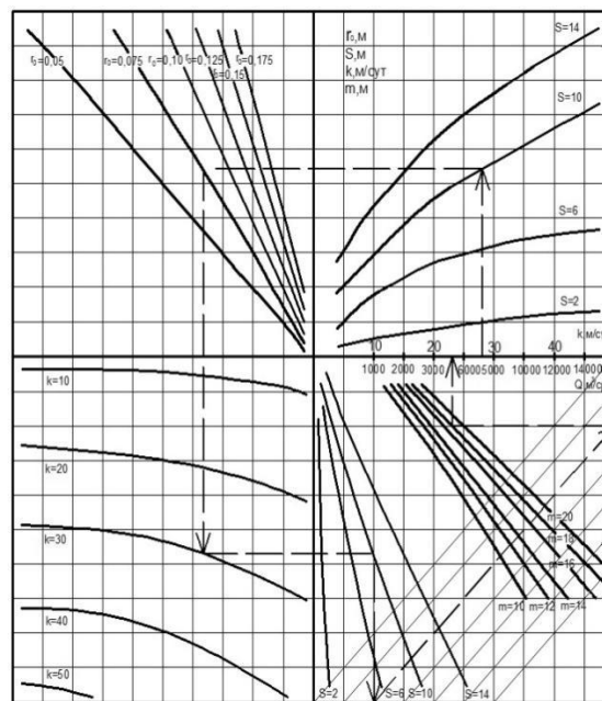
Рис.5 Номограмма для определения величины производительности совершенных вертикальных колодцев в напорных водоносных слоях / The nomogram to determine the performance of perfect vertical wells in pressure aquifers
