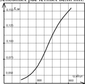
Рис.3. График влияния радиуса колодца на его производительность /Graph radius well effect on its performance
