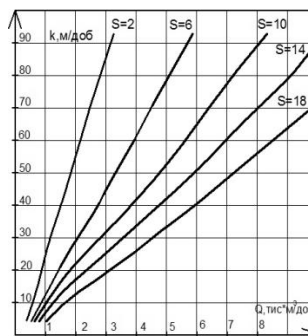
Рис.4. График влияния величин коэффициента фильтрации водоносного слоя и снижения уровня воды в колодце на его производительность /
