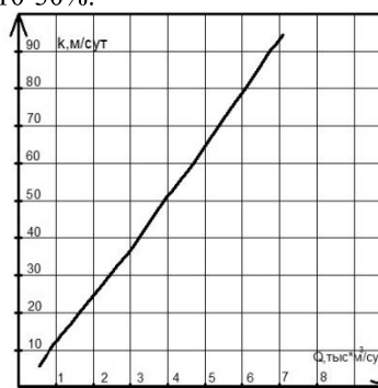
Рис.1. График влияния коэффициента фильтрации водоносного слоя на производительность колодца / Schedule influence the filtration coefficient of the aquifer on the performance of the well
