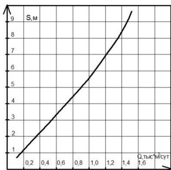
Рис.2. График влияния величин снижения уровня воды в колодце на его производительность /
