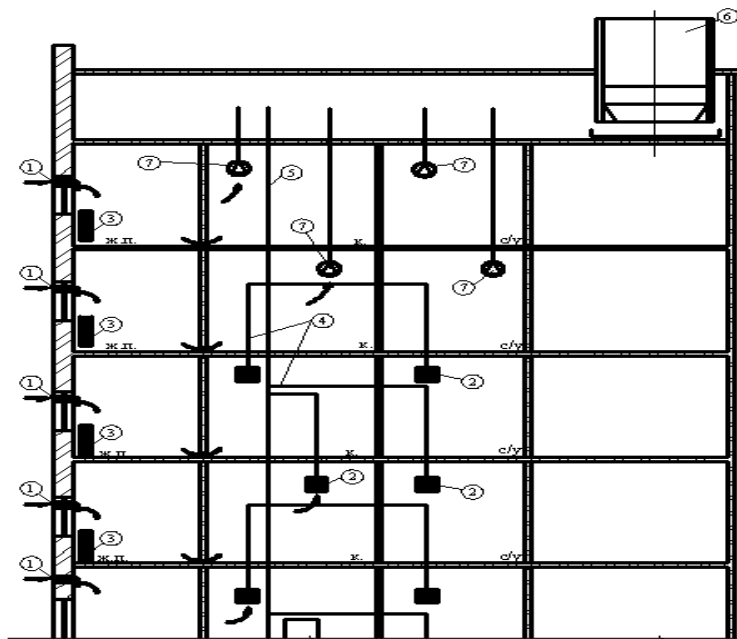
Рис. 1 Схема системы естественной вентиляции с отдельными и общим сборным вытяжным каналом в здании с теплым чердаком/
